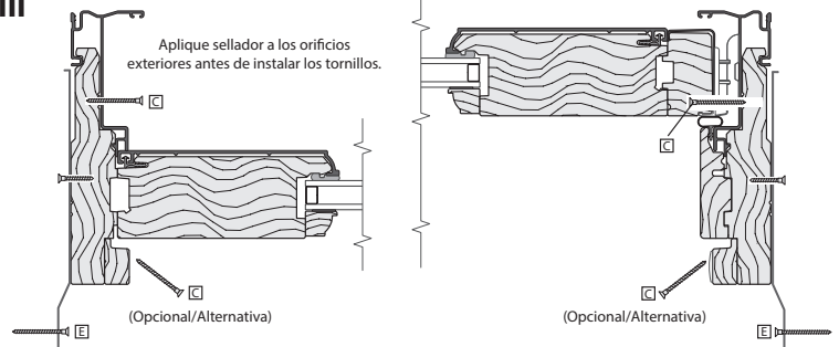
Sujetador/tornillo, jambas
