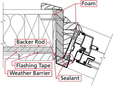
JAMB - 2 X 4 Frame
