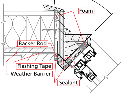
JAMB - 2 X 4 Frame
