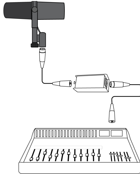
Configuración del preamplificador
