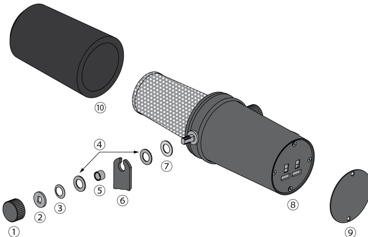
Conjunto de montaje: vista de despiece
