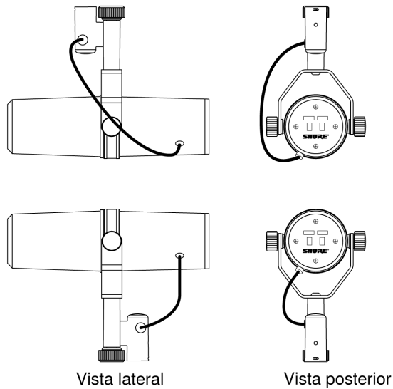
Configuración de montaje en pedestales tipo jirafa y de micrófono
