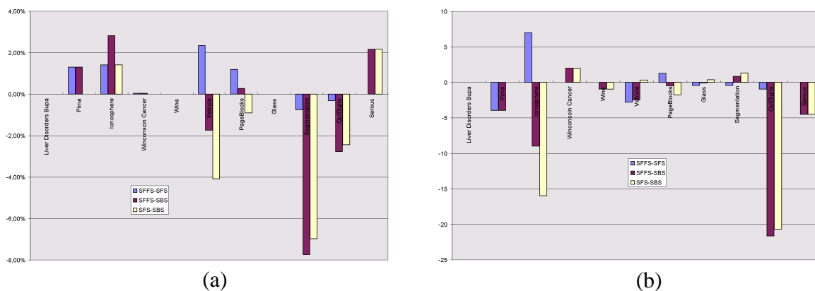
Figure 17. Ecarts entre les différentes méthodes utilisant l'approche wrapper pour le taux de reconnaissance global de l'architecture (a) et le nombre d'attributs moyen employé par chaque réseau (b).
