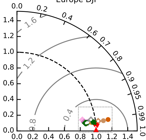
Europe DJF
