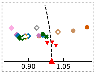
Europe DJF
