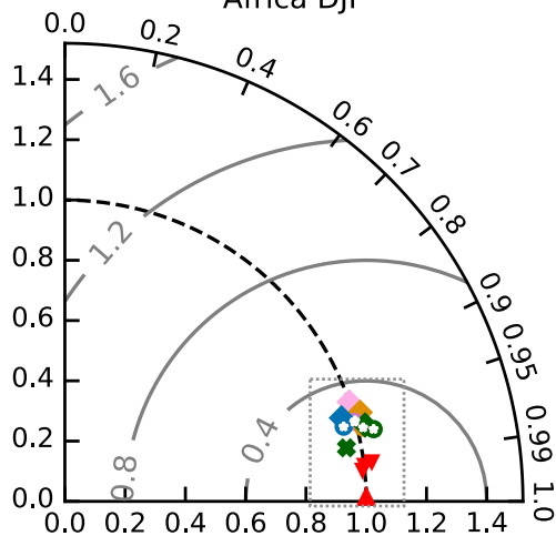
Africa DJF
