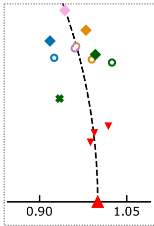
Africa DJF
