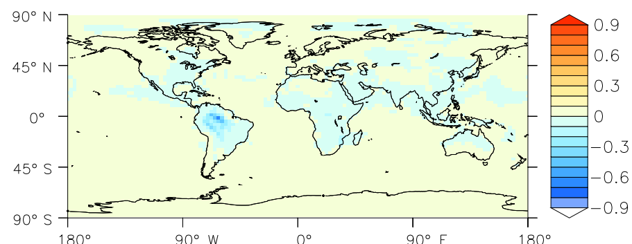
(d) POLY-FULL: isoprene difference (nmol mol -1 )
