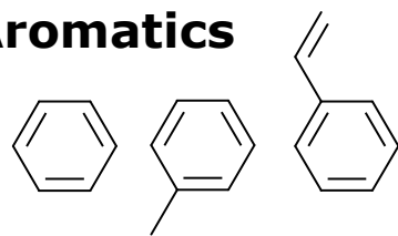
Benzene Toluene Styrene
