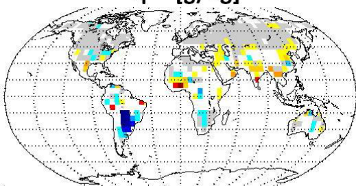
c) |MERRA-2 - Had| - |MERRA - Had| q^{2m} [g/kg]
