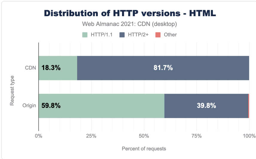
図21.13. HTML（デスクトップ）用HTTPバージョンの配布。
