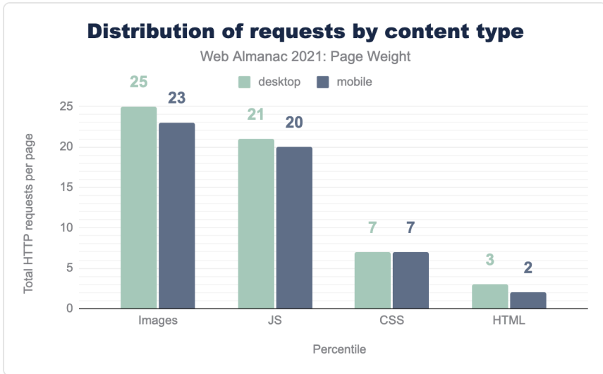
図19.5. コンテンツタイプ別のリクエスト数の中央値。
