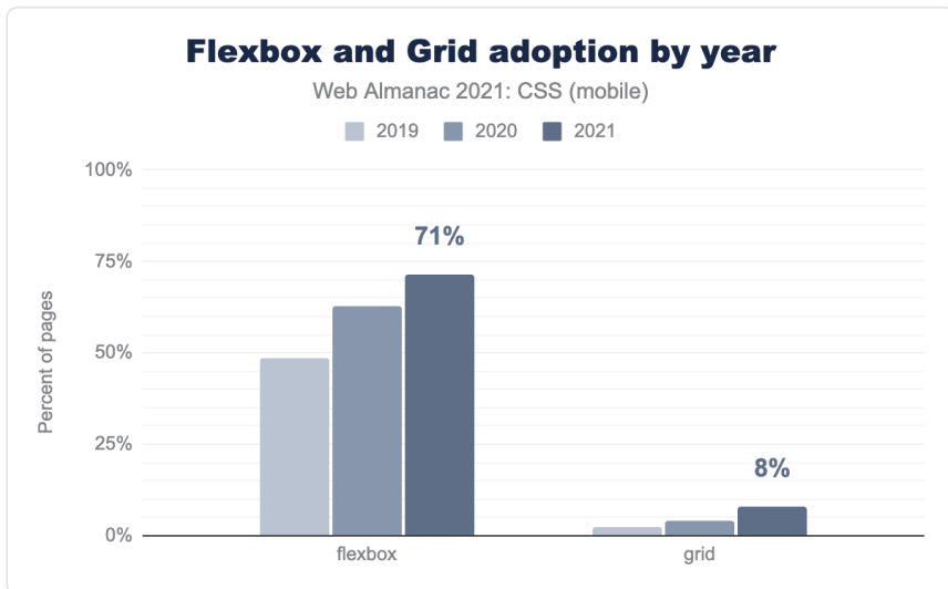
図1.36. モバイルデバイスでのFlexboxおよびGridレイアウトの採用。
