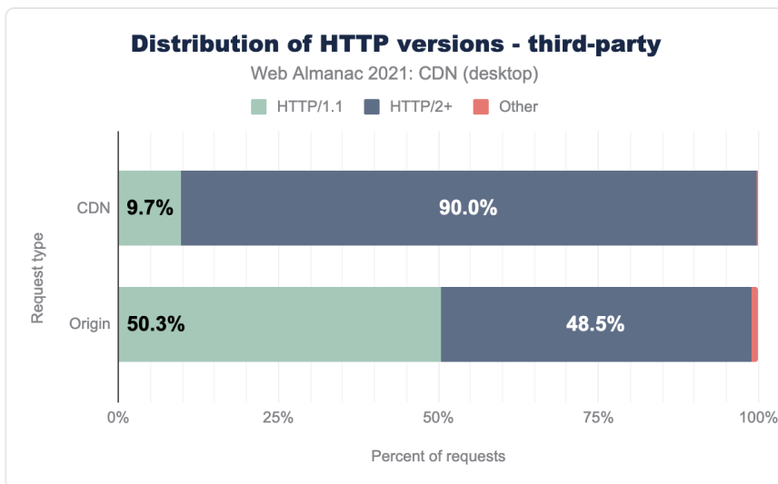
図21.15. サードパーティリクエスト用HTTPバージョンの配布（デスクトップ）。
