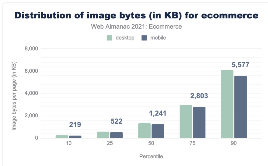
図17.23. eコマース向け画像バイトの配布
