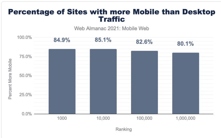
図13.2. デスクトップよりモバイルのトラフィックが多いサイトの割合。
