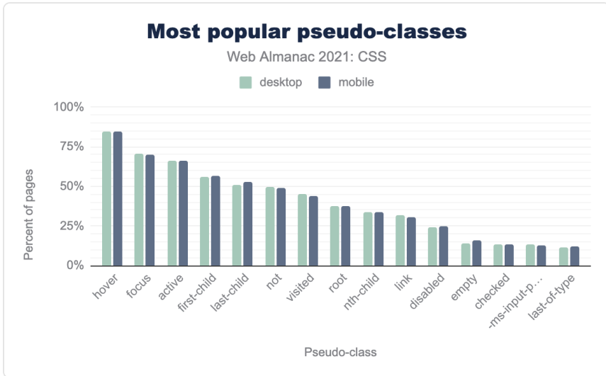
図1.9. もっともポピュラーな疑似クラスです。
