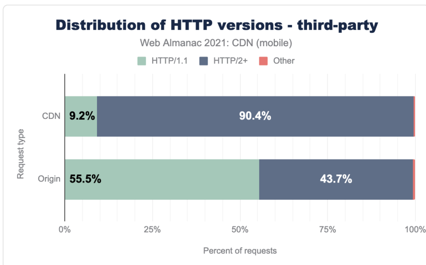
図21.16. サードパーティからのリクエストに対応したHTTPバージョンの配布（モバイル）。
