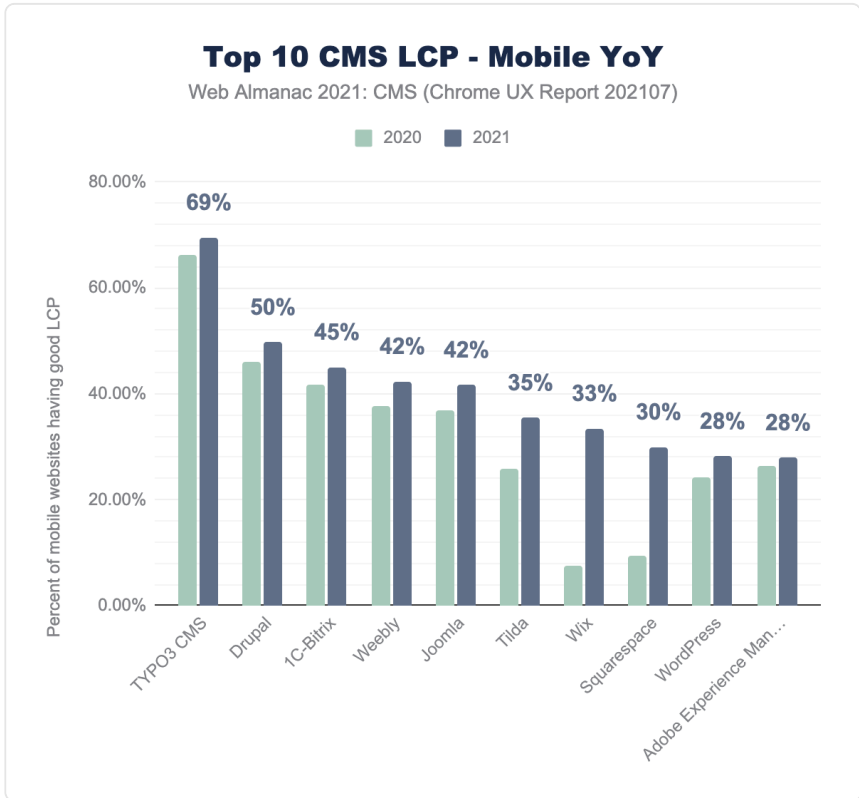
図16.11. CMS上位10社のモバイルビューのLCPパフォーマンス前年比。
