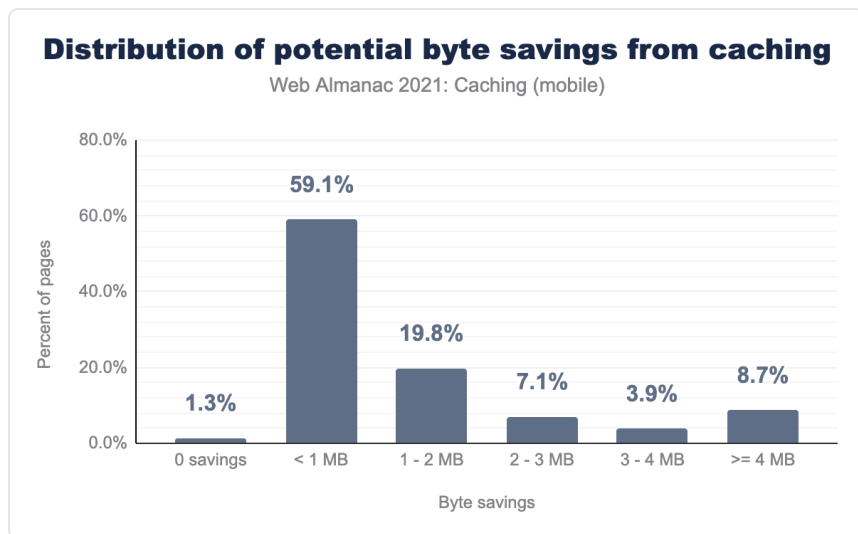
図23.21. キャッシュによる潜在的なバイト数削減の分布。
