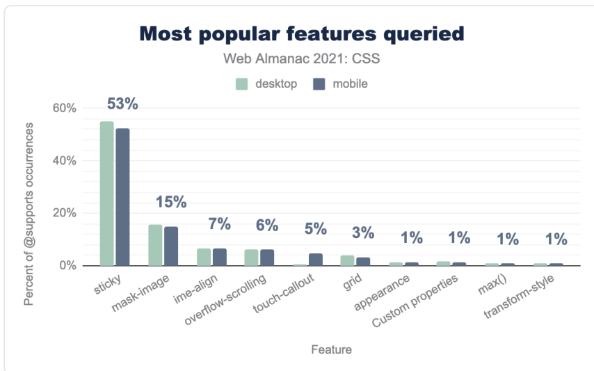
図1.47. CSSの代表的な機能を @supports で照会できます。
