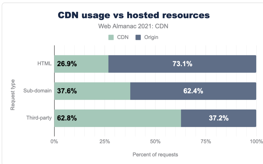
図21.1. CDNの使用とホスティングされたリソースの比較。
