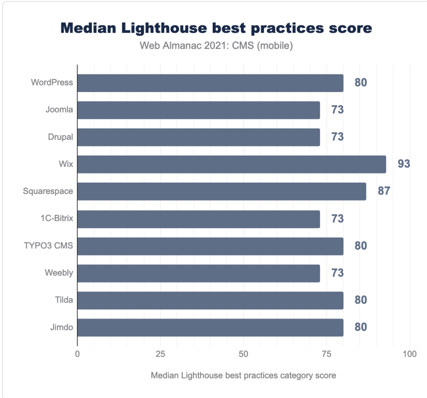
図16.19. CMS上位10社のライトハウスベストプラクティススコア中央値。
