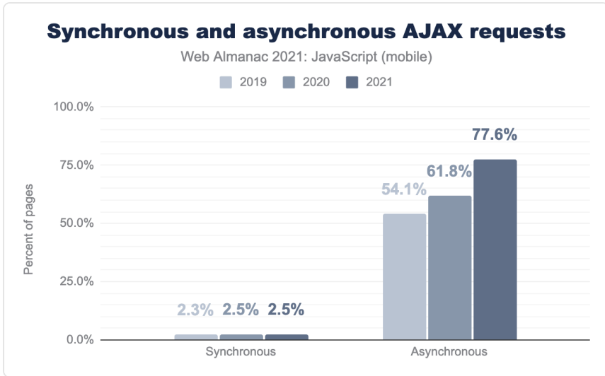
図2.32. 長年にわたる同期および非同期AJAXリクエストの使用状況。
