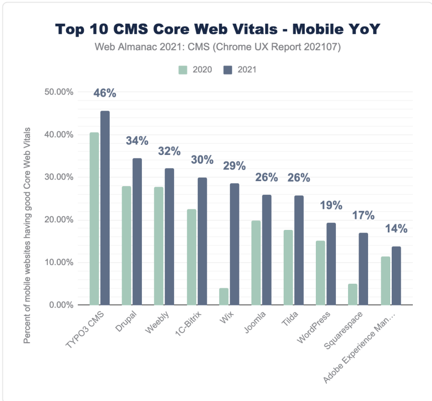
図16.9. トップ10 CMSコアWebバイタルのモバイルビューのパフォーマンス前年比。
