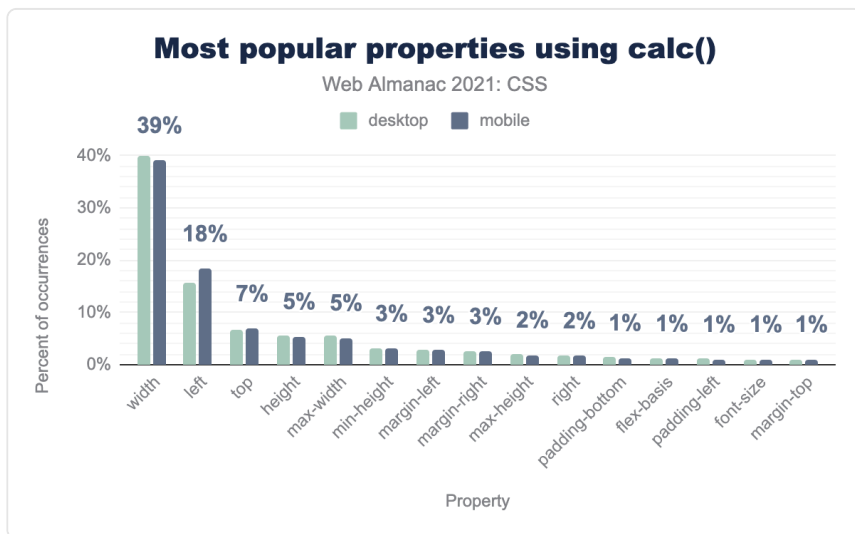
図1.18. calc() 関数を使った代表的なプロパティです。
