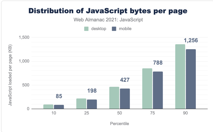
図2.1. ページごとに読み込まれるJavaScriptの量の分布。
