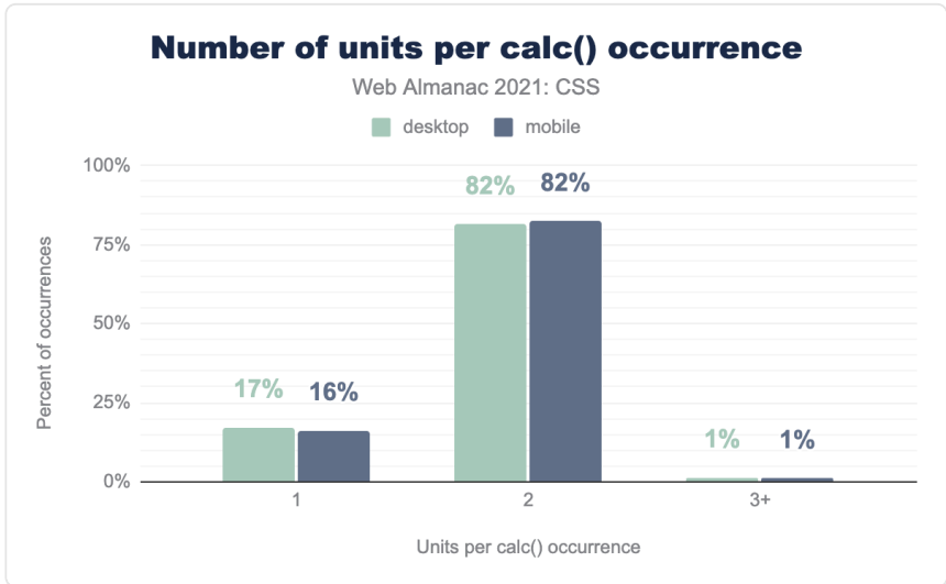
図1.21. 関数 calc() で使用されるユニークなユニットの数です。
