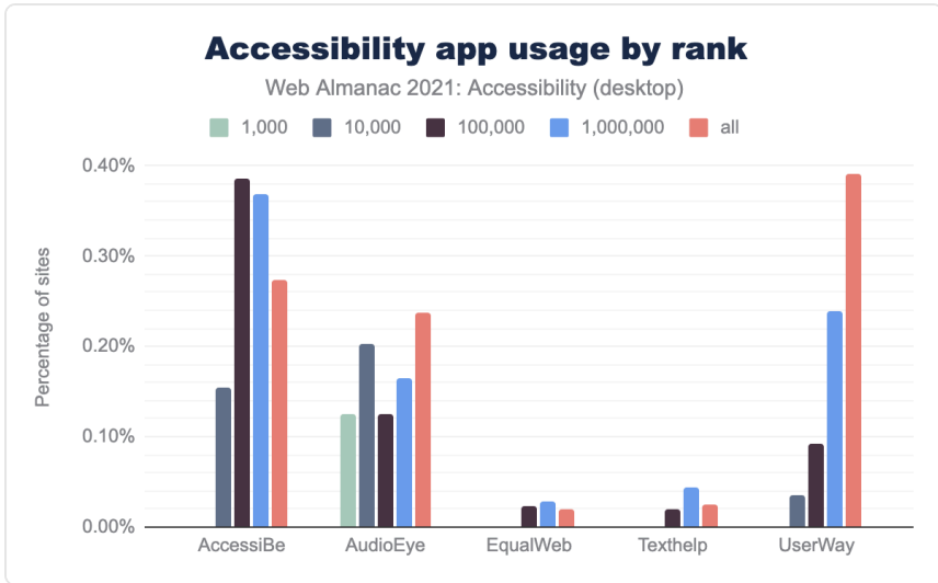
図9.30. アクセシビリティ・アプリのランク別利用状況。
