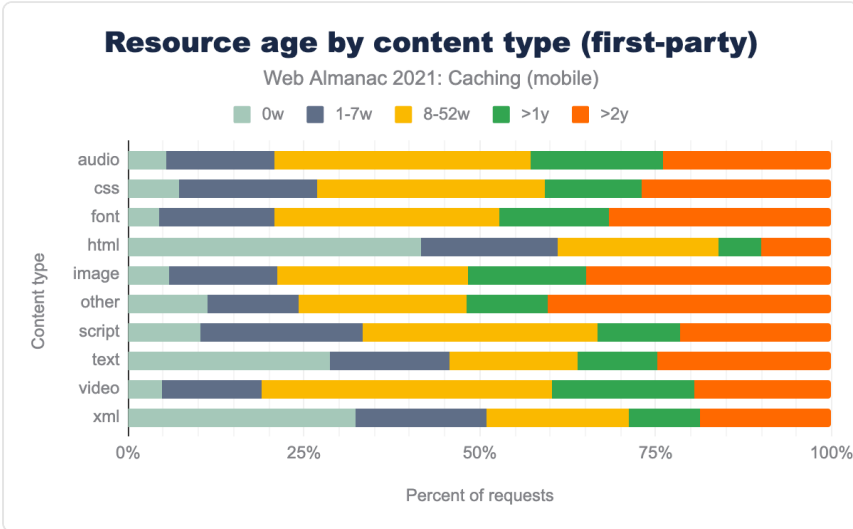
図23.16. コンテンツタイプ別のファーストパーティリソースエイジの分布（モバイルのみ）。
