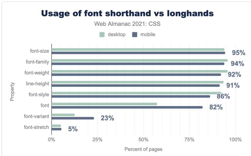
図1.59. よく使われるフォントのプロパティ
