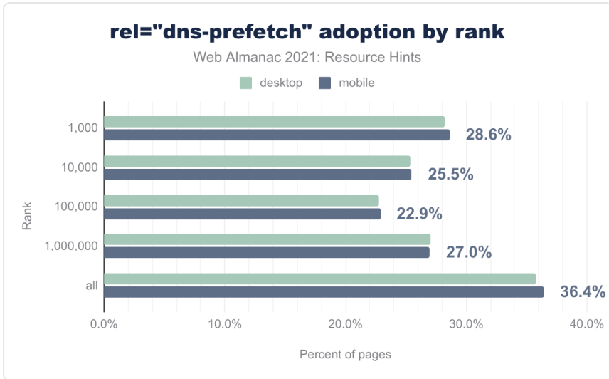
図20.4. rel="dns-prefetch" の採用状況をCrUXランクで区分したものの。
