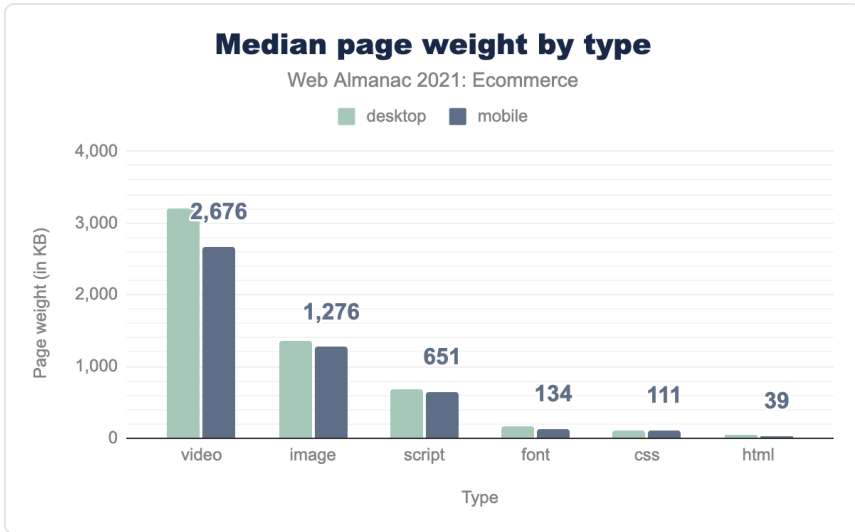
図17.19. タイプ別ページキロバイトの中央値。
