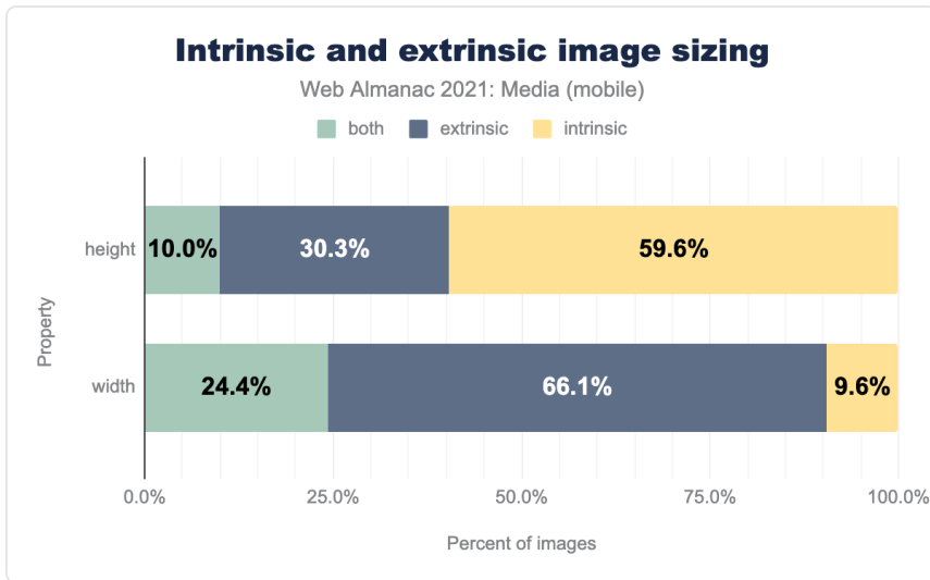
図5.24. 内在的および外在的な画像サイズ調整。
