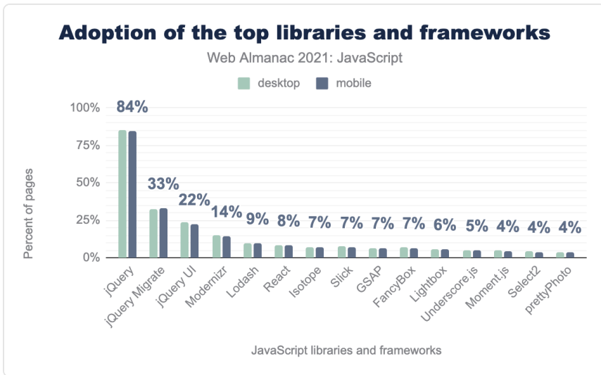
図2.25. JavaScriptのライブラリやフレームワークの使用状況。
