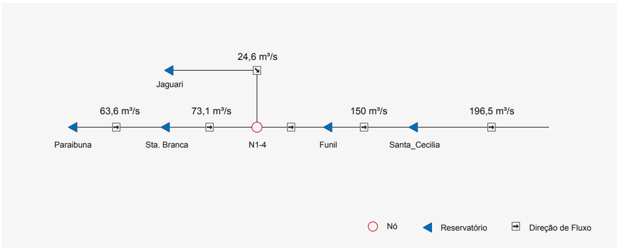
Figura 4.12 – Diagrama com a vazão regularizada pelas hidrelétricas do rio Paraíba do Sul
