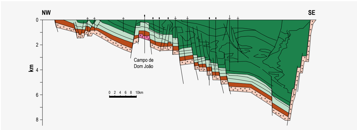
Figura 5.9 – Perfil geológico da Bacia Sedimentar do Recôncavo (Fonte: PETROBRAS)
