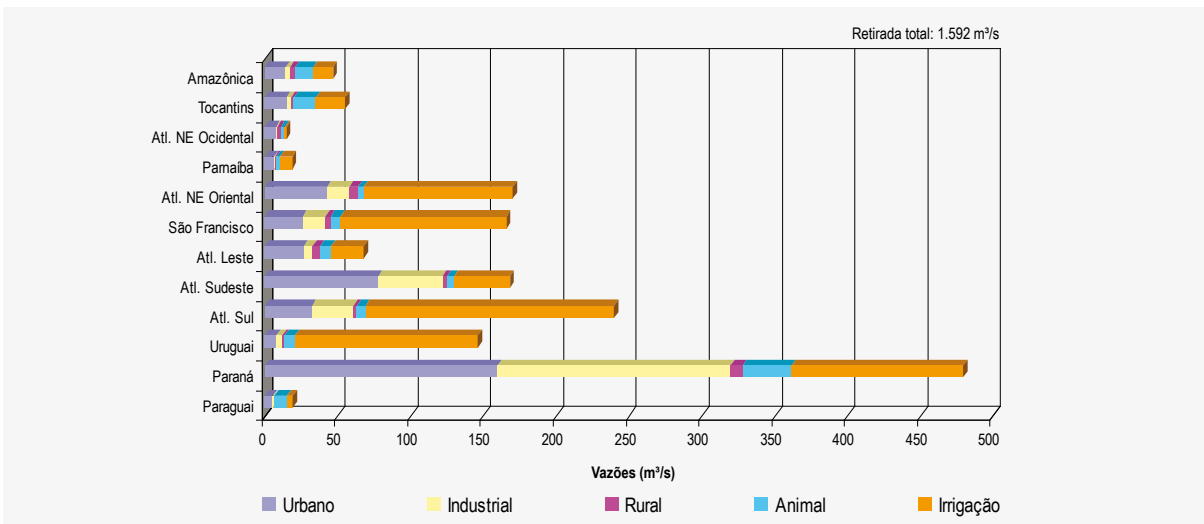
Figura 6.2 – Vazões de retirada para os diferentes usos nas regiões hidrográficas
