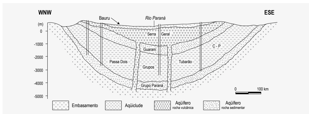
Figura 5.11 – Perfil geológico da Bacia Sedimentar do Paraná. Os sistemas aquíferos Furnas e Ponta Grossa pertencem ao Grupo Paraná (Fonte: Modificado de REBOUÇAS, 1988)
