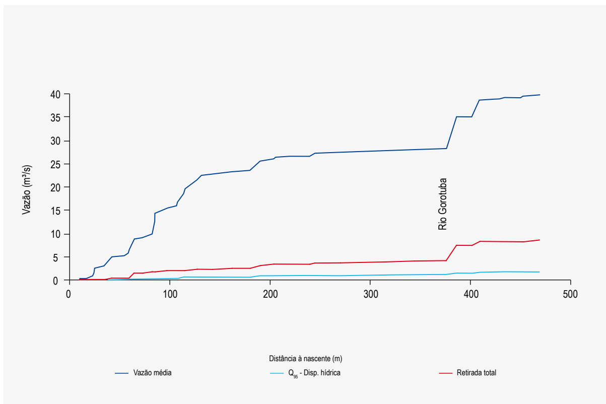
Figura 8.2 – Disponibilidade e demanda de recursos hídricos, ao longo do rio Verde Grande
