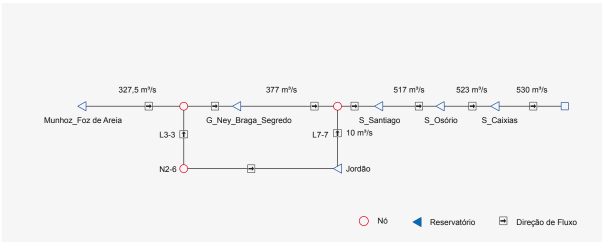
Figura 4.18 – Diagrama com a vazão regularizada pelas hidrelétricas do rio Iguaçu
