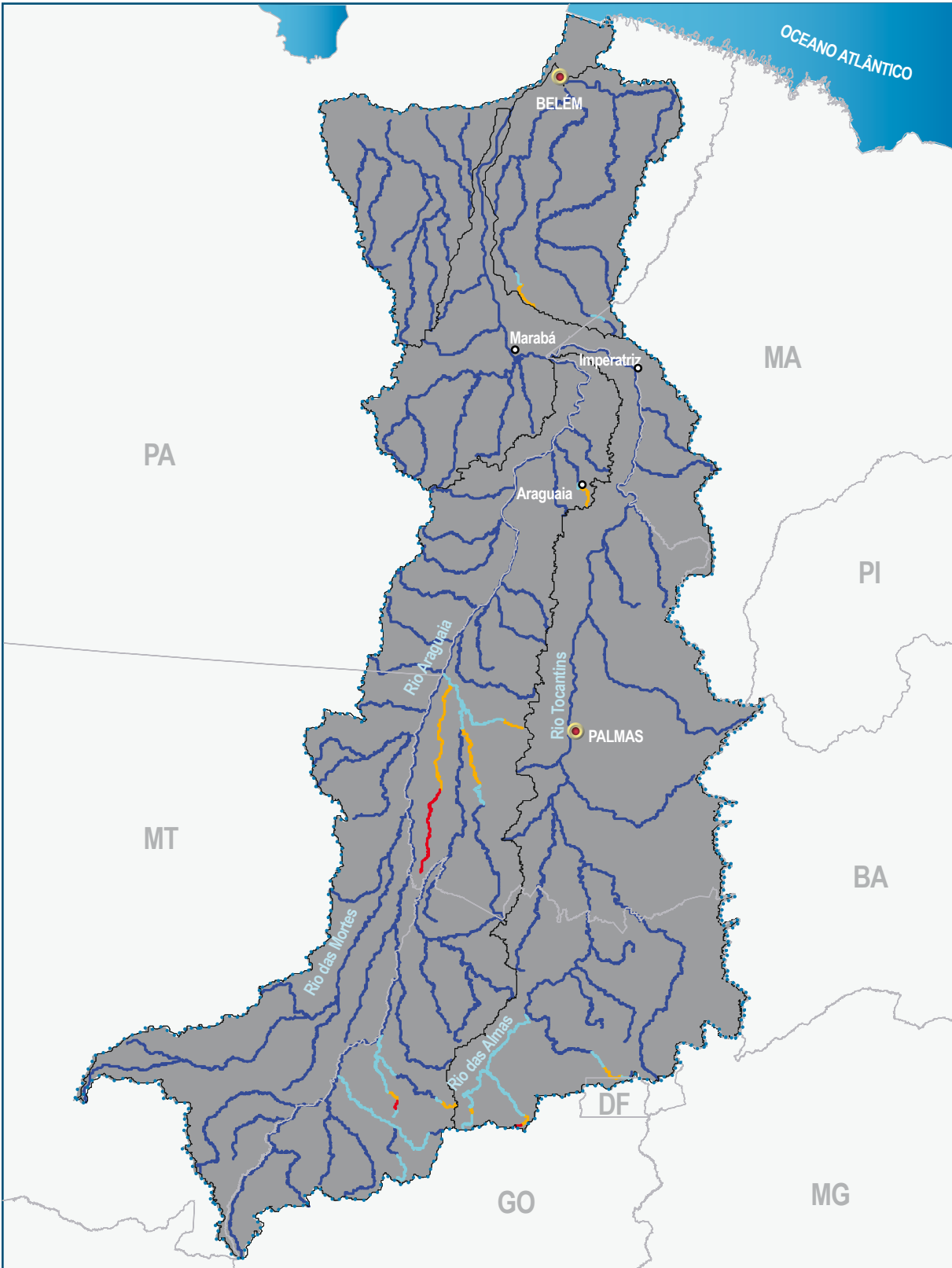
Figura 8.8 – Relação entre Demanda e Disponibilidade Hídrica na Região Hidrográfica Tocantins–Araguaia
