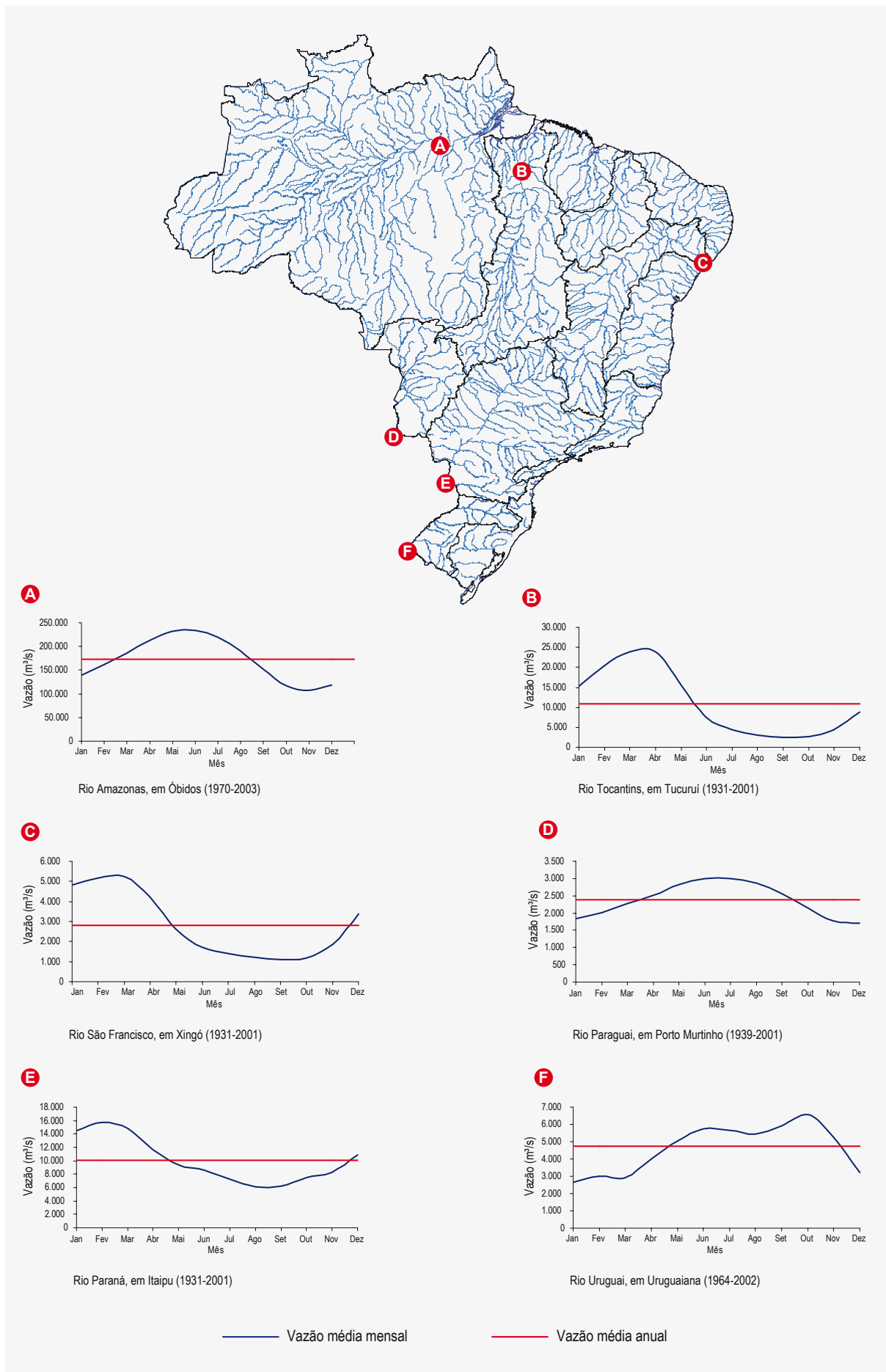
Figura 4.8 – Hidrogramas nas regiões hidrográficas Amazônica, Tocantins/Araguaia, São Francisco, Paraná, Paraguai e Uruguai
