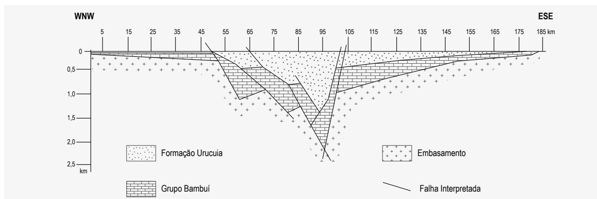
Figura 5.10 – Perfil gravimétrico interpretado, a sul da cidade de Barreiras-BA (Fonte: Adaptado de BOMFIM; GOMES 2004)
