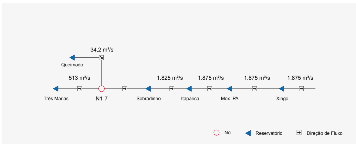
Figura 4.11 – Diagrama com a vazão regularizada pelas hidrelétricas do rio São Francisco
