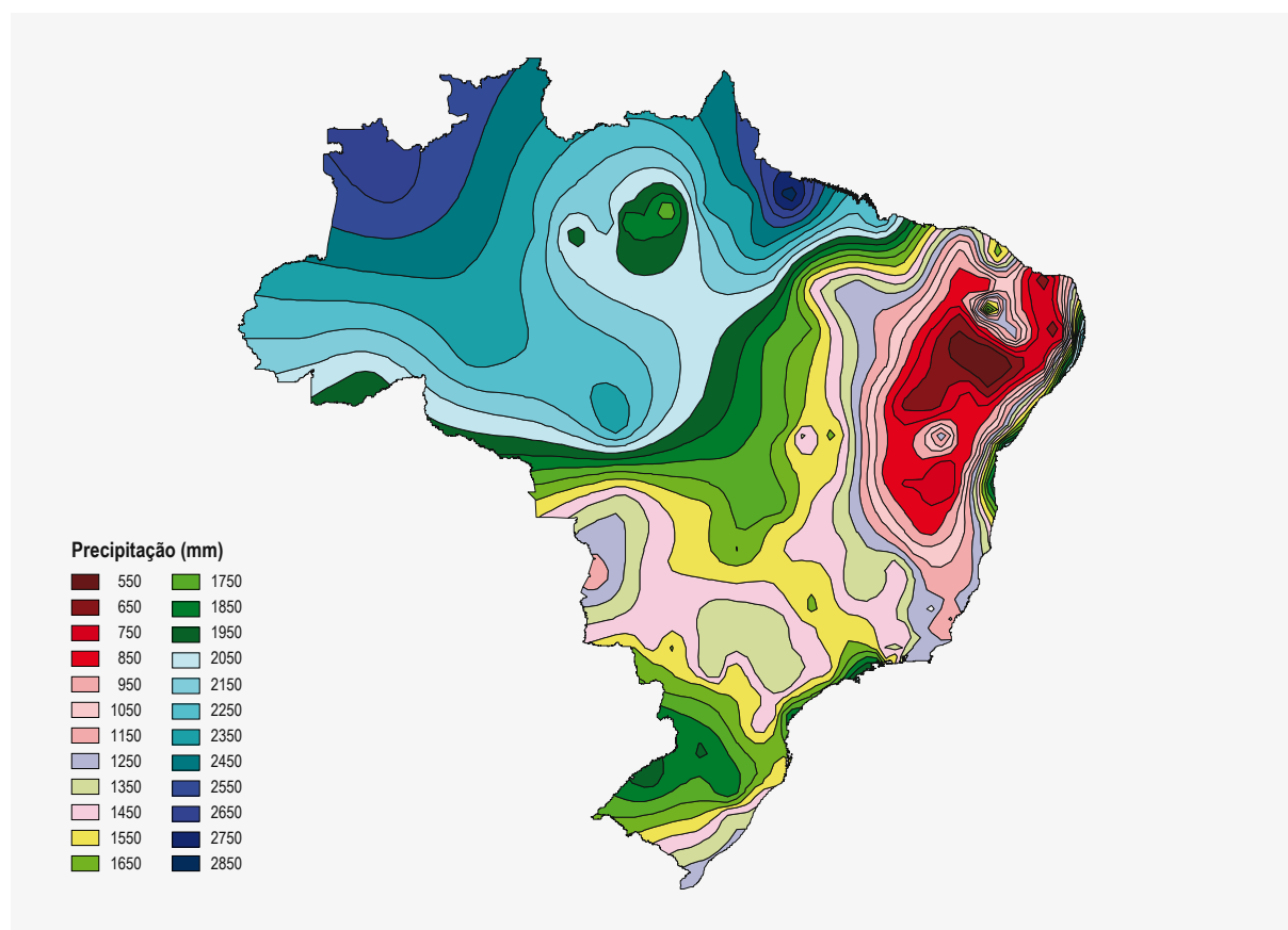
Figura 4.1 – Isoietas anuais no País, entre 1961 e 1990
