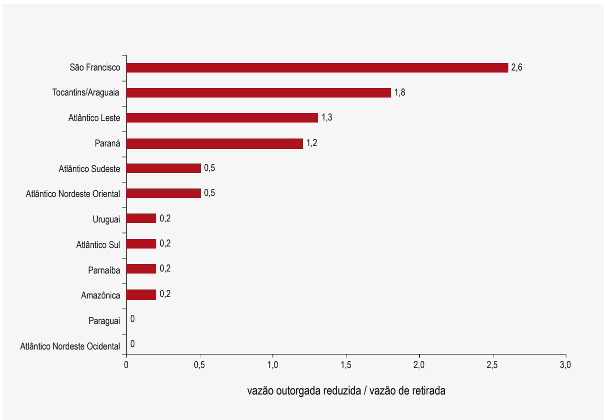
Figura 7.6 – Relação entre a vazão outorgada (reduzida) e a vazão de retirada nas regiões hidrográficas
