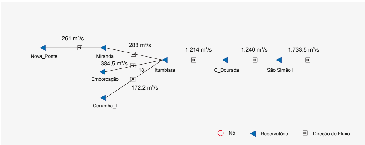
Figura 4.13 – Diagrama com a vazão regularizada pelas hidrelétricas do rio Paranaíba
