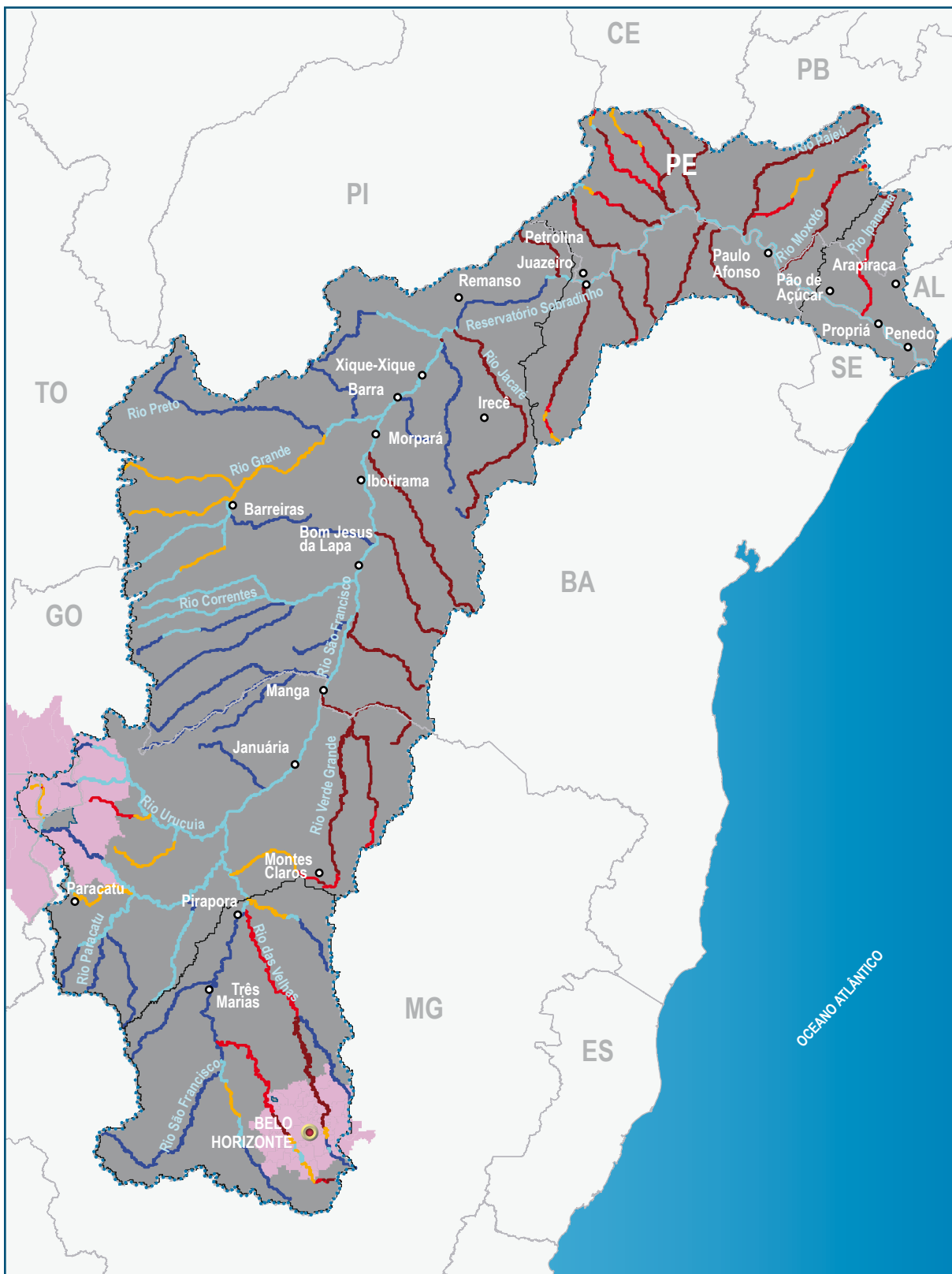
Figura 8.13 – Relação entre Demanda e Disponibilidade Hídrica na Região Hidrográfica São Francisco
