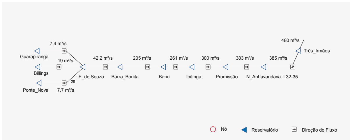
Figura 4.15 – Diagrama com a vazão regularizada pelas hidrelétricas do rio Tietê
