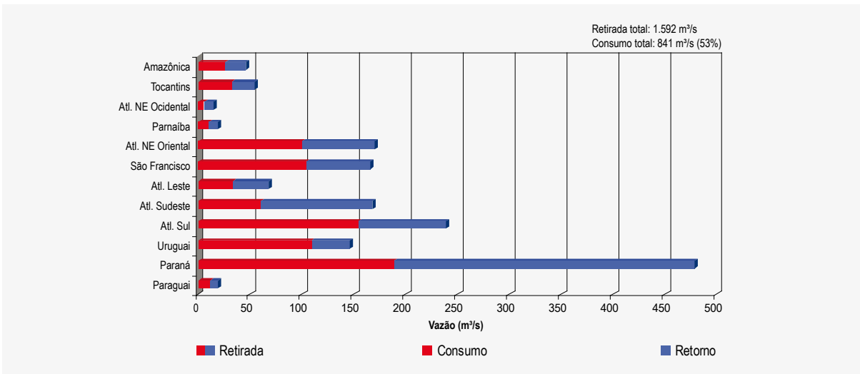
Figura 6.1 – Vazões de retirada, consumo e retorno nas regiões hidrográficas
