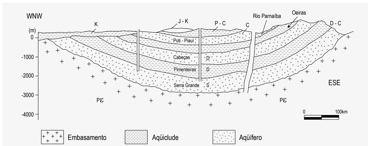
Figura 5.5 – Perfil geológico na Bacia Sedimentar do Parnaíba (Fonte: Modificado de REBOUÇAS, 1988)
