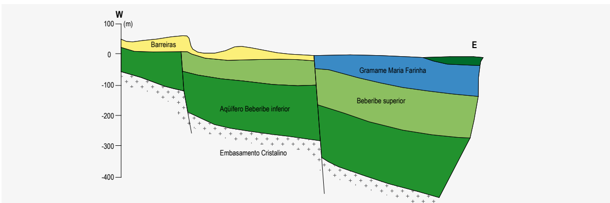
Figura 5.8 – Perfil geológico na zona norte de Recife-PE (Fonte: Adaptado de OLIVEIRA, 2003, por MANOEL FILHO, 2004)
