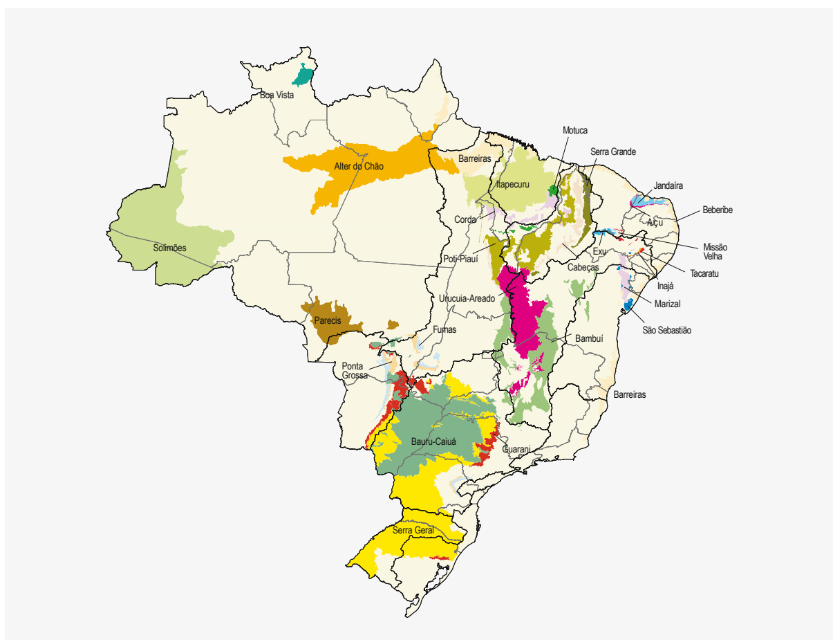
Figura 5.2 – Área de recarga dos principais sistemas aquíferos do País
