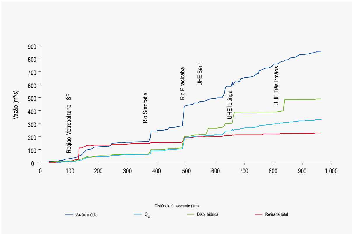
Figura 8.4 – Disponibilidade e demanda de recursos hídricos, ao longo do rio Tietê
