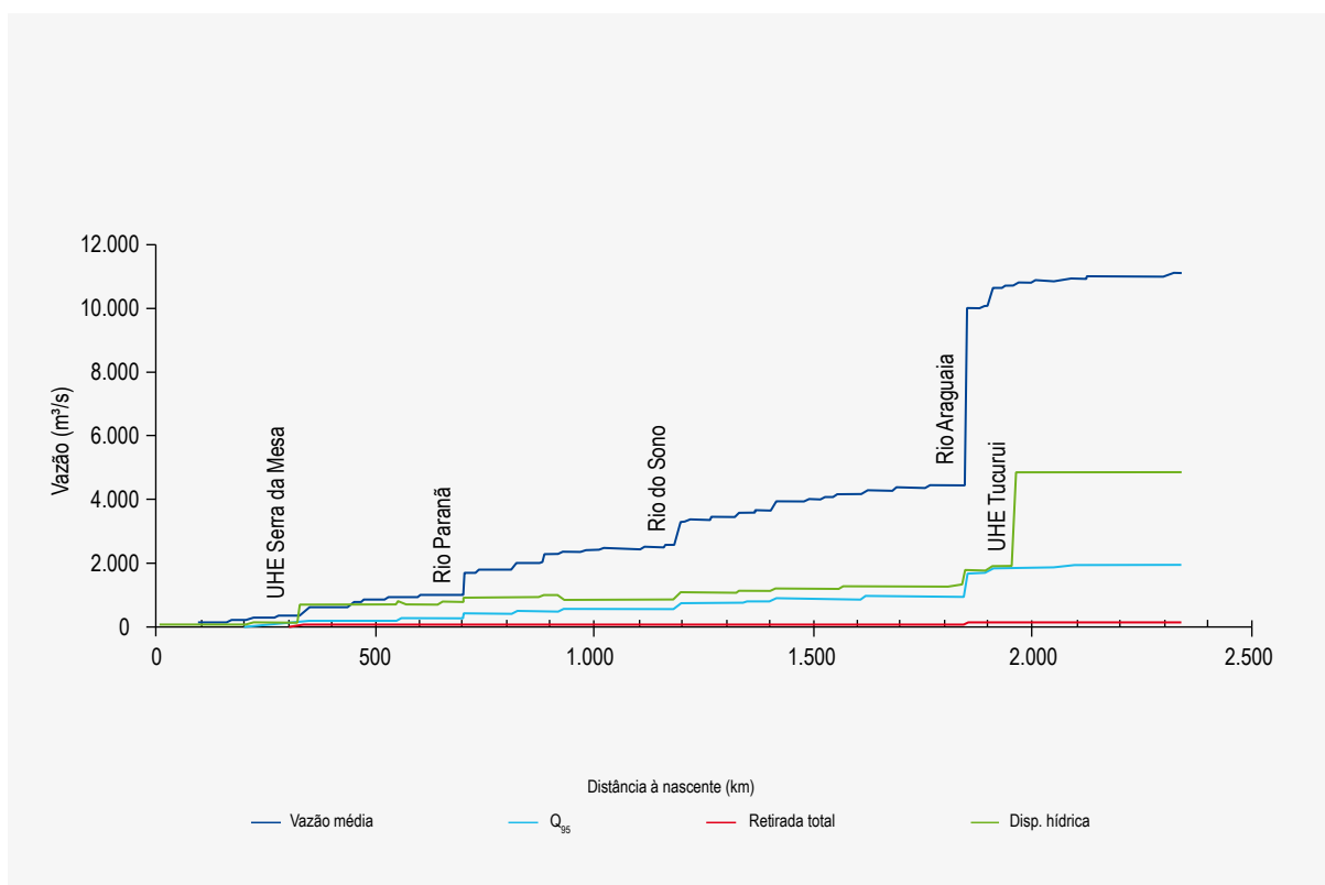
Figura 8.3 – Disponibilidade e demanda de recursos hídricos, ao longo do rio Jaguaribe
