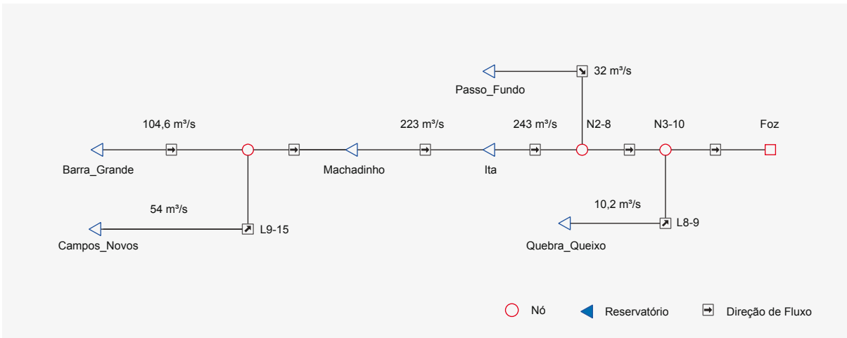
Figura 4.19 – Diagrama com a vazão regularizada pelas hidrelétricas do rio Uruguai
