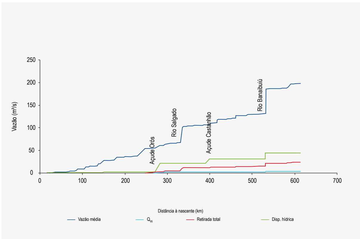
Figura 8.5 – Disponibilidade e demanda de recursos hídricos, ao longo do rio Tocantins
