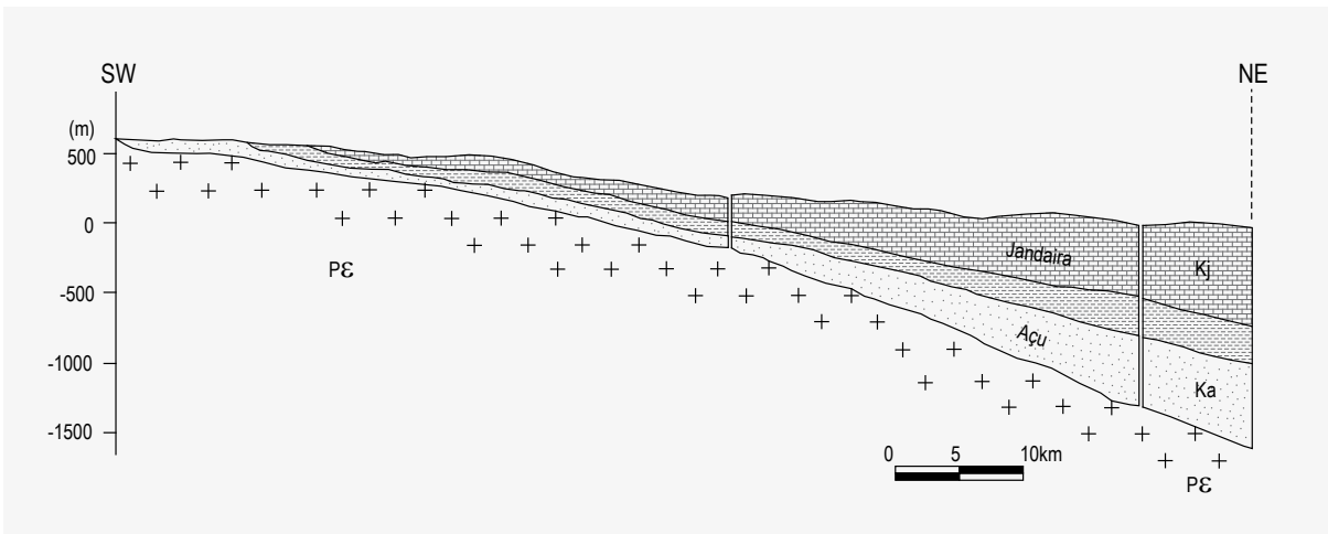
Figura 5.4 – Perfil geológico da Bacia Potiguar (Fonte: Modificado de REBOUÇAS, 1988)
