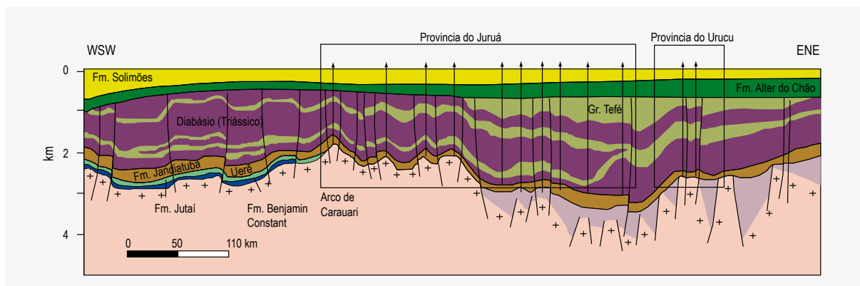
Figura 5.3 – Perfil geológico na Bacia Sedimentar do Amazonas (Fonte: PETROBRAS)
