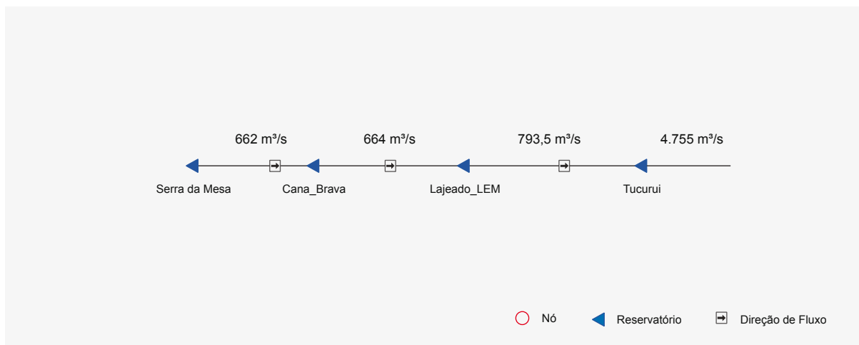
Figura 4.10 – Diagrama com a vazão regularizada pelas hidrelétricas do rio Tocantins
