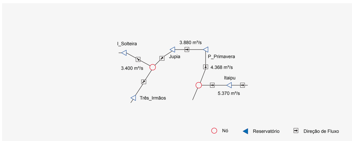
Figura 4.17 – Diagrama com a vazão regularizada pelas hidrelétricas do rio Paraná
