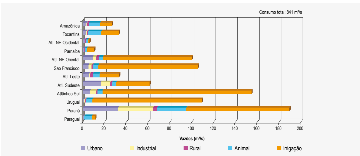
Figura 6.3 – Vazões de consumo para os diferentes usos nas regiões hidrográficas
