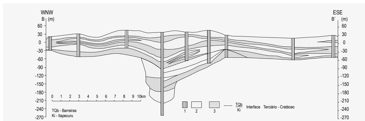
Figura 5.6 – Perfil geológico próximo a São Luís-MA (Fonte: SOUSA, 2004)
