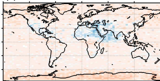
(d) Clean continental
