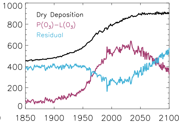
CESM2-WACCM
