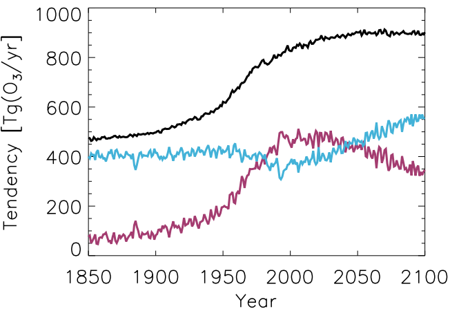
GFDL-ESM4
