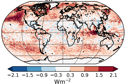
(d) ORG: \Delta AIE_{SW} avg = 0.39 \text{ Wm}^{-2}
