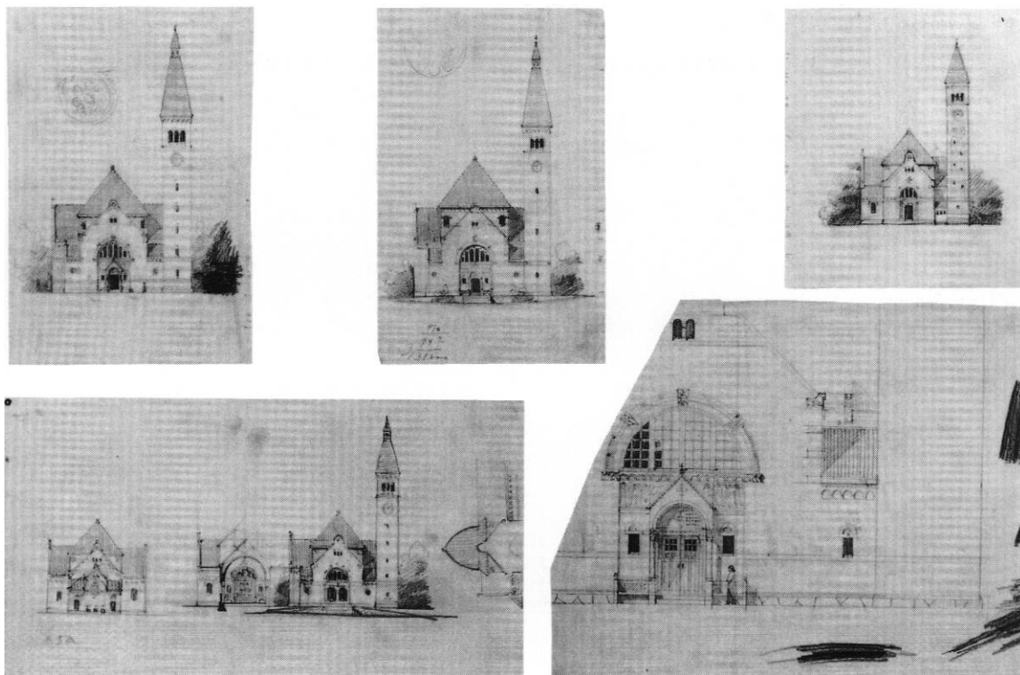
Fig. 13. Udkast til kirkebygningen tegnet i foråret 1900 af Niels Jacobsen (s. 1591). I menighedsrådets arkiv. - Proposal for the church building drawn in the spring of 1900 by Niels Jacobsen.
