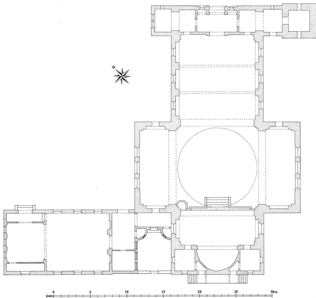
Fig. 2. Plan 1:300. Tegnet og suppleret af MN 1998 på grundlag af tegninger i Stadsarkivet og NM. - Plan.
