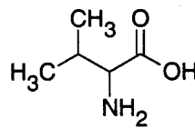
Valine (Val)
