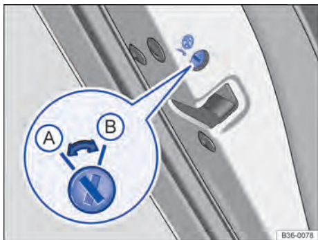
Fig. 10 Na porta traseira esquerda: trava de segurança para crianças (A) desligada, (B) ligada.
