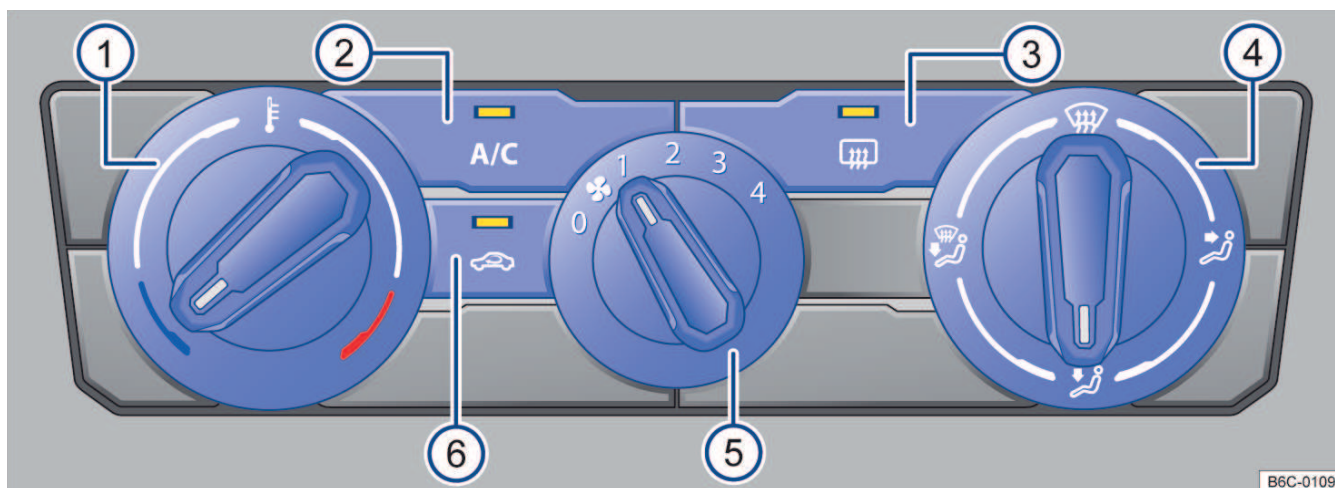
Fig. 84 Comandos do ar-condicionado.
