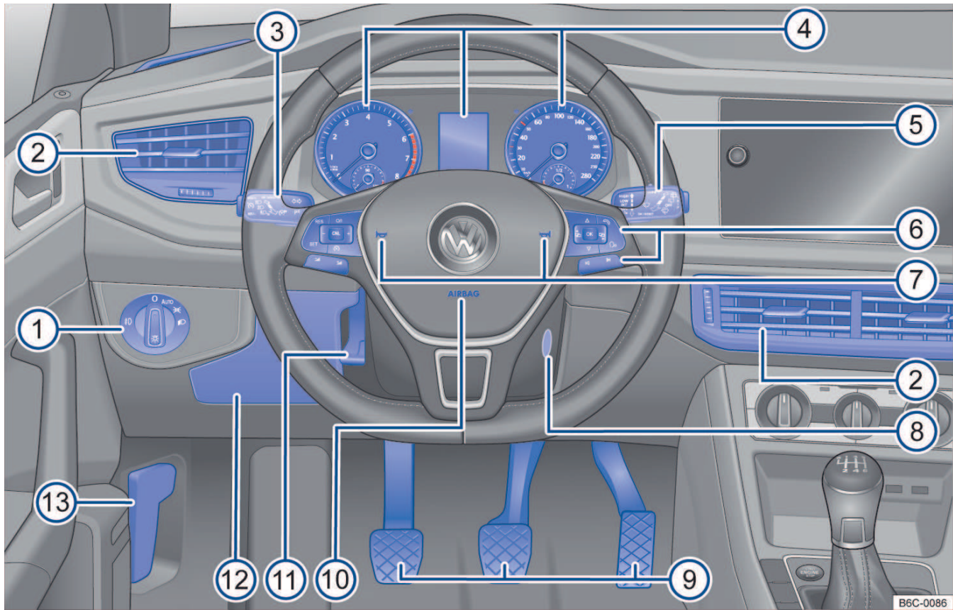
Fig. 5 Vista geral do lado do condutor.
