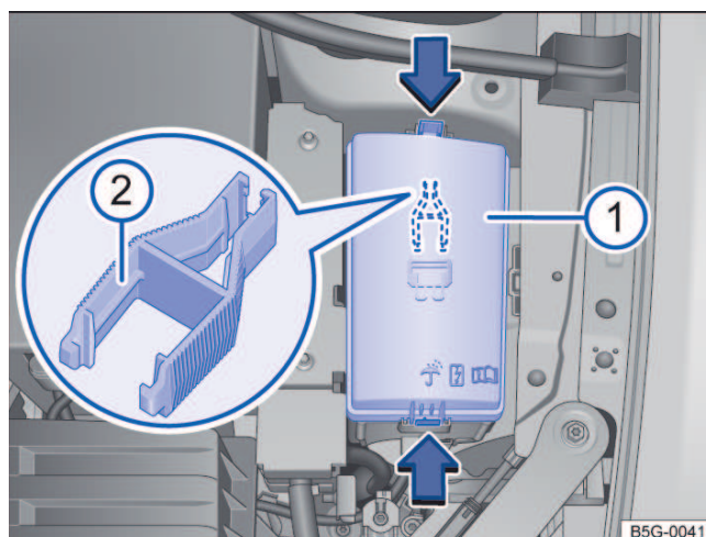
Fig. 140 No compartimento do motor: cobertura ① da caixa de fusíveis com pinça de plástico ②.
