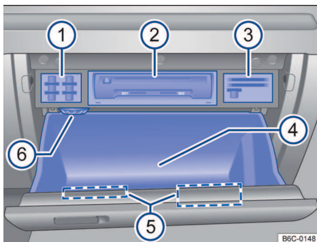
Fig. 109 No lado do passageiro dianteiro: porta-luvas aberto.
