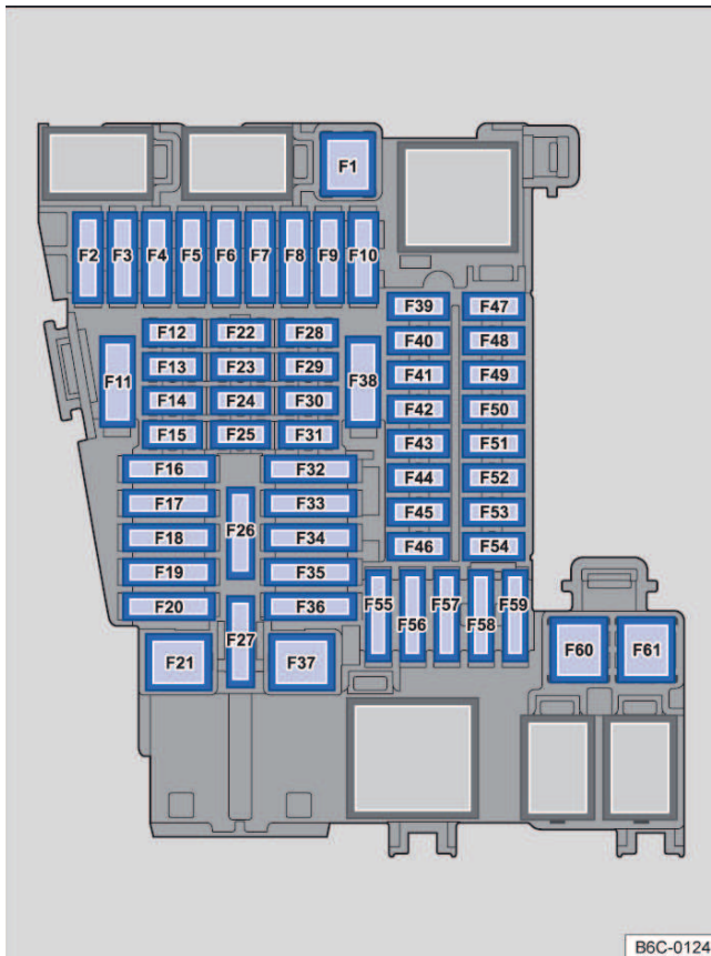
Fig. 141 No painel de instrumentos: disposição dos fusíveis.
