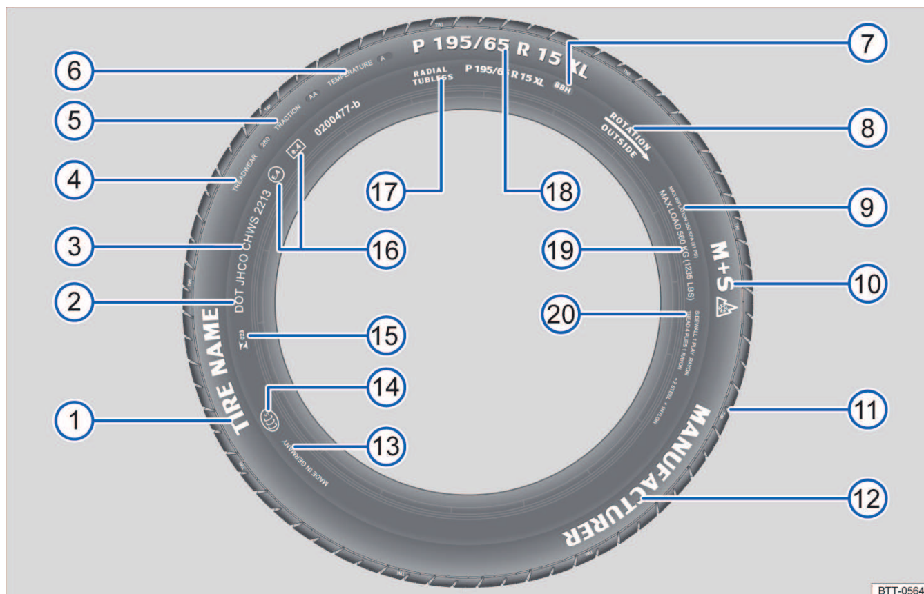
Fig. 163 Inscrição dos pneus internacional (exemplo).
