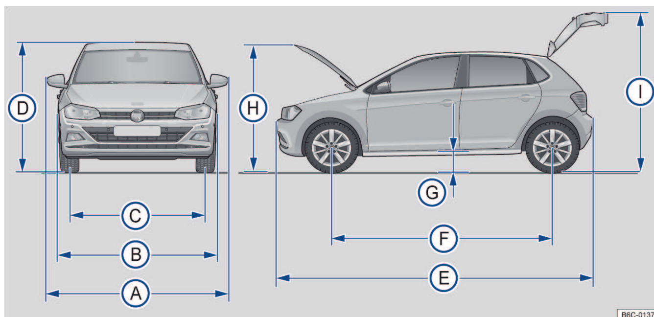
Fig. 176 Dimensões.
