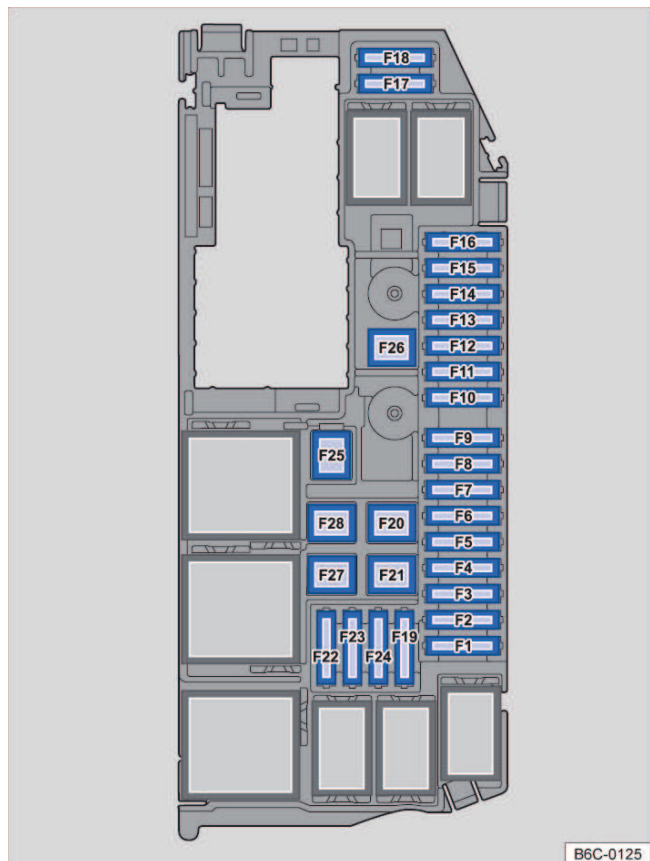
Fig. 142 No compartimento do motor: disposição dos fusíveis.
