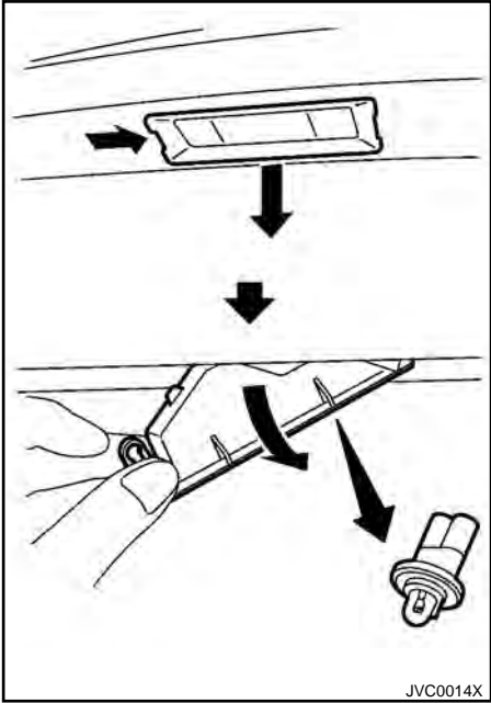
Luz da placa de licença traseira
