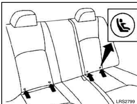
Localizações dos pontos de ancoragens inferiores do sistema ISOFIX/LATCH (se equipado)
