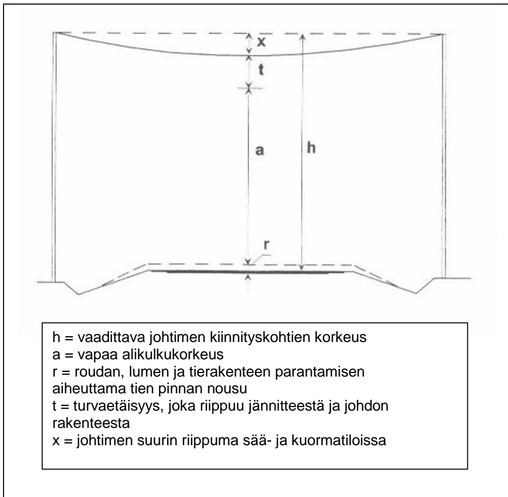
Kuva 5.34 Tien kanssa risteävien ilmajohtojen asennuskorkeuteen vaikuttavat tekijät (TIEH 2001a, s. 17).
