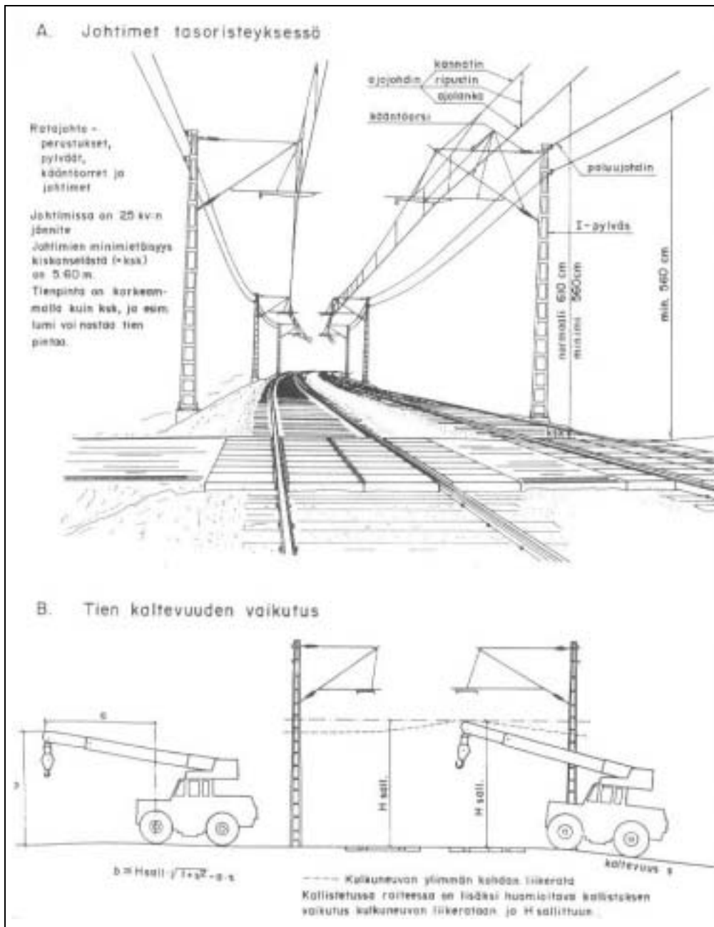
Kuva 5.32 Sähköistetyn radan johtimien huomioon ottaminen erikoiskuljetuksissa (TIEL 1992a, liite 7).
