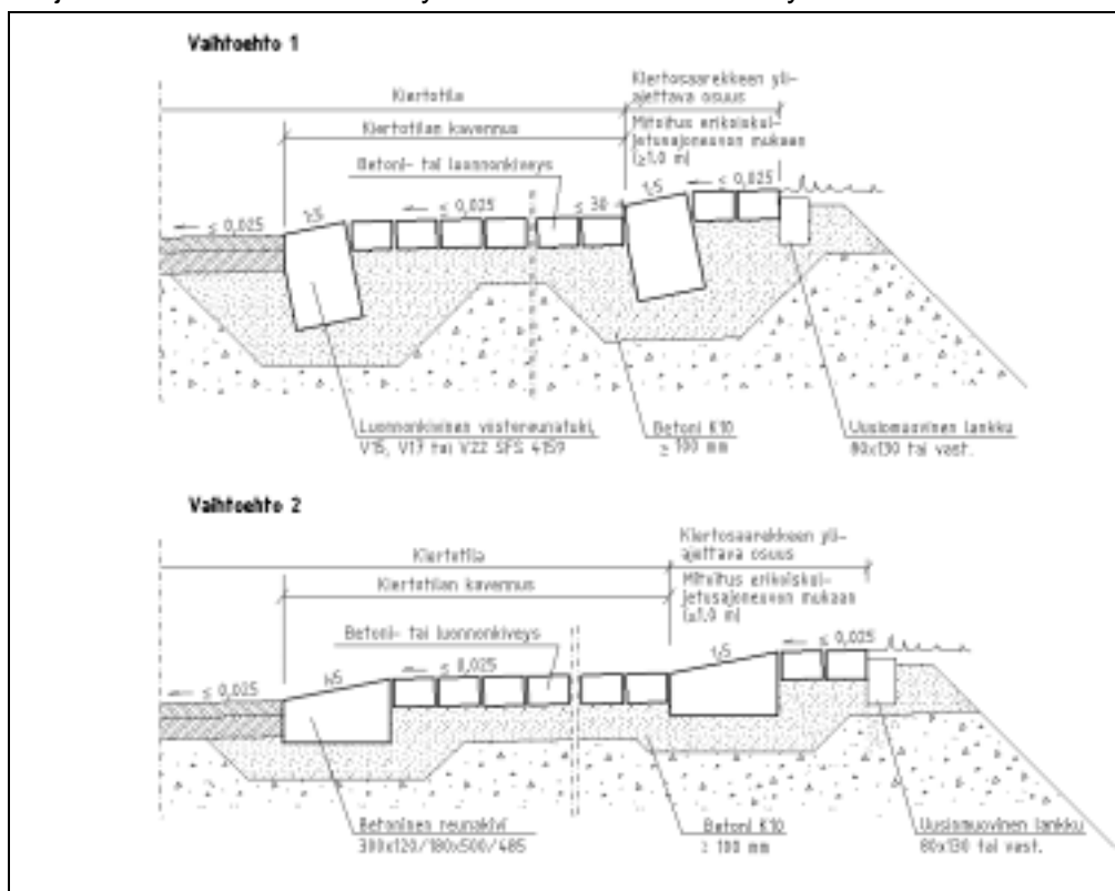
Kuva 5.4 Kiertotilan kaventaminen betoni- ja luonnonkiveyksellä (TIEH 2001b, s. 76).
