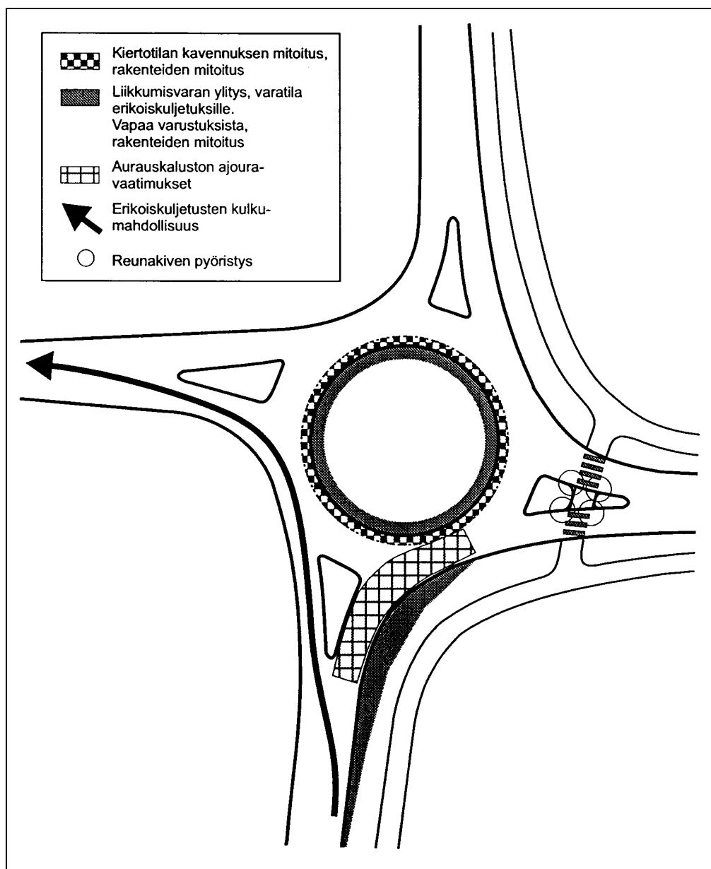
Kuva 5.6 Erikoiskuljetusten vaatimat järjestelyt kiertoliittymässä (TIEH 2001b, s. 80).
