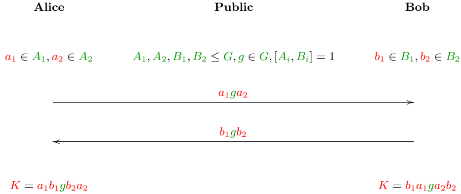
Fig. 5. The Double Coset KEP
