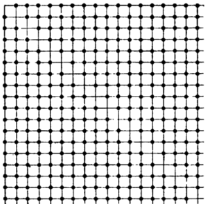
Fig. 7. Matrix von 0'.
