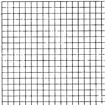
Fig. 5. Matrix von 0.
