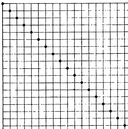
Fig. 6. Matrix von 1'.
