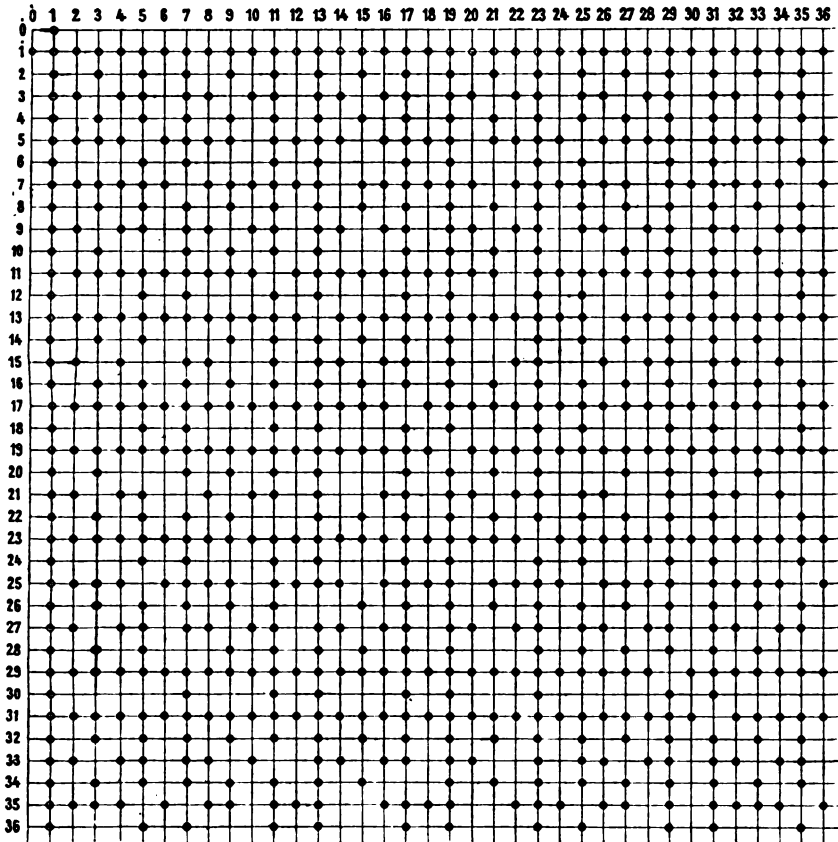
Fig. 3. Matrix des Relativa: „teilerfremd mit-“.
