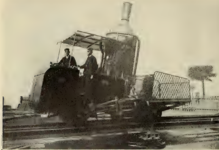
Première locomotive à crémaillère, système Riggenbach (type primitif de la locomotive du chemin de fer Vitznau-Rigi) 1871.
