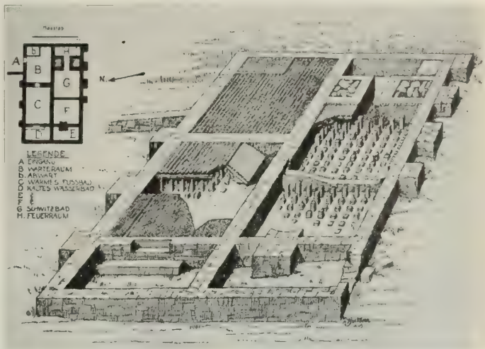
Thurgovie. Plan des bains romains d'Eschenz. D'après Keller et Reinert : Urgeschichte des Thurgaus.
