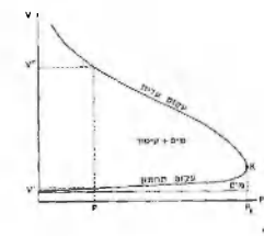
ציור 1: אידוי מים בתנאים קבועים ייגום, עומק הרתחה — הנפת כספי-הרתחה. עומק עליון — נפת רפסודר. תנאים בין שני התנאים הוא ש"ה שתי גודל מים — איזובר; מתחילת נמצא תחום רמים, ופעולה תחום הקיטור היחיד.
