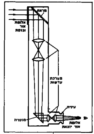
סכמה של פריסקופ
