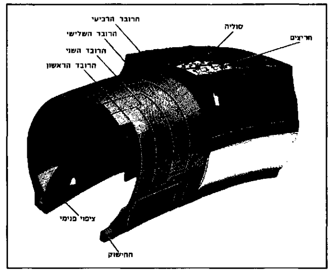
כמה צמיג נוסעים — 4 רבדים — ללא אבוב
