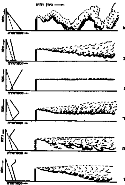
ציור 2: פיזור המזהמים מארובה במסלול סמפרטורה שונים. הרוח הממוצעת נושבת משמאל לימין. הקו המדוסט מתאר ספל סמפרטורה של 10^{\circ}\text{C}/\text{km} . תנאים טובים לפיזור קיימים כאשר יש אינוורסיה מסוג לקרקע (מתחת לארובה הפולסת) וירידה מהירה של הטמפרטורה מעל הארובה (מצב ד'). במסלול הסמפרטורה חלש על יד הקרקע ויש אינוורסיה ברום (מצב טיפוסית לחדשי הקיץ בישראל). נלכדים המזהמים בניו בסמים האינוורסיה לקרקע (מצב ו')
