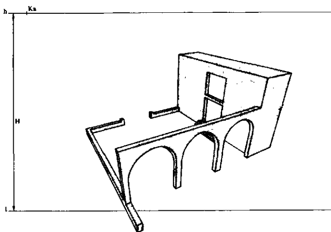
סוגי הפרספקטיווה. מלמעלה למטה: לוח הפרספקטיווה מאונך למישור התומך אך משופע לגבי הדפנות האנכיים של הבניין. לוח הפרספקטיווה מאונך למישור התומך ומקביל לקיר הקשתות של הבניין. לוח הפרספקטיווה סיווה משופע לגבי המישור התומך וגם לגבי הדפנות האנכיים של הבניין. H— קו האופק; I— ציר הפרספקטיווה; H— גובה העין; K— נקודת המנון (נקודת הכינוס)
