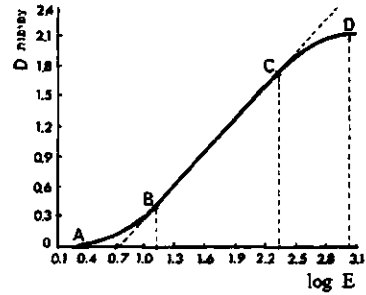
עקומה אפיינית של סרט צילום, המתארת את היחס בין הצפיפות (D) והחשיפה (E); נתונה כסולם לוגאריטמי. באיור B-C צפיפויות הנטיב הן ביחס ישר ללוגריתם בהירויות הנושא המצולם; A-B - איזור, תת חשיפה; C-D - חשיפת יתר.
