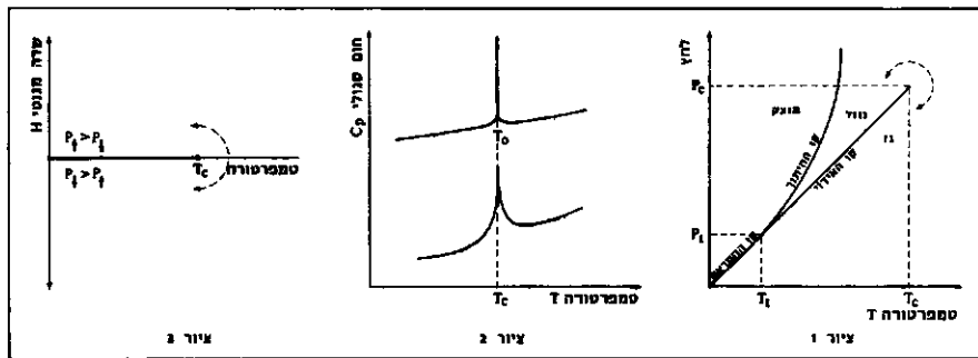
ציור 1: דיאגרמת הפנות של מים; ציור 2: השתנות החום הסגולי עם הטמפרטורה במעבר מסדר ראשון (בגרה תחתון) ובמעבר מסדר שני (בגרה העליון); ציור 3: מעבר פנות מנטני
