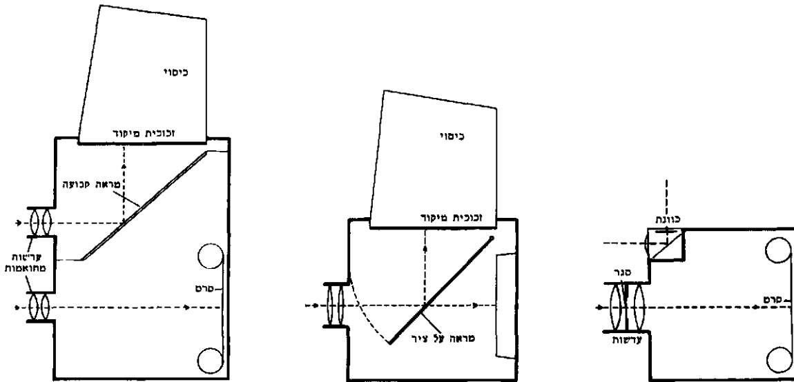
מהלך הקרניים במצלמות שונות. מימין לשמאל: סכמה של מצלמה עם כוונת; סכמה של מצלמת רפלקס; סכמה של מצלמת רפלקס בפולת עדשות
