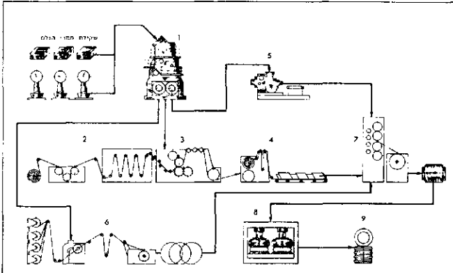
שלבי הייצור של צמיגים
