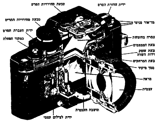
חתך במצלמת רפלקס חדשה (פינולטה XM)
