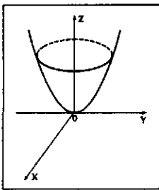
פרבולואיד סיבובי
