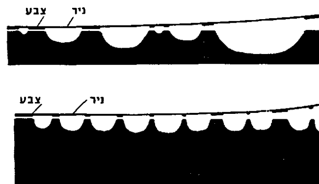
טעולה: חתך של גלופת קו (הגדלה 800%); טמטה: חתך של גלופת רשת (הגדלה 600%)
