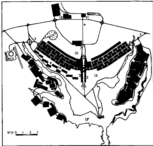
תכנית העיר ברזיליה, בירת ברזיל — עיר חדשה, שהוקמה לפי תכנית מוכנה, ושמשש דוגמה לכינוי ערים מונומנטליות ולהמחשת הארדיכלות בימינו. העיר תוכננה ע"י לוסיו קוסטה, ורוב בנייניה הציבוריים הוקמו ע"פ תכניותיו של הארדיכל א. ניסיאר (ע"ש). שני ציורי-תחבורה יוצרים את שלד המבנה העירוני: א. ציר מונומנטלי ראשי; ב. ציר ראשי כאוורי המגורים (תמ'); ע"ע ברזיליה, כרך סילוואים 1. כיכר 3 הרשויות; 2. משרדי הממשלה; 3. קתדראלה; 4. מרכזי-תרבות; 5. מרכז לספרה ולתחבורה; 6. מנדל הסלנוויזיה; 7. בית-העיריה; 8. מגורים בצפיפות נכונה; 9. מגורים בצפיפות נמוכה; 10. ספורט; 11. תחנת-רפת; 12. תעשייה; 13. נמל-תעופה; 14. שגרירויות; 15. אוניברסיטה; 16. ארמון הנשיא; 17. אגם פלאטות
