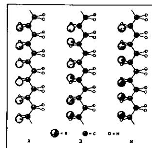
ציור 5: מבנה מרחבי של פולימרים ויניליים. (א) אטקטי; (ב) סינדריו; (ג) איזוטקטי (שים לב למקום הסיפון השמאלי)
