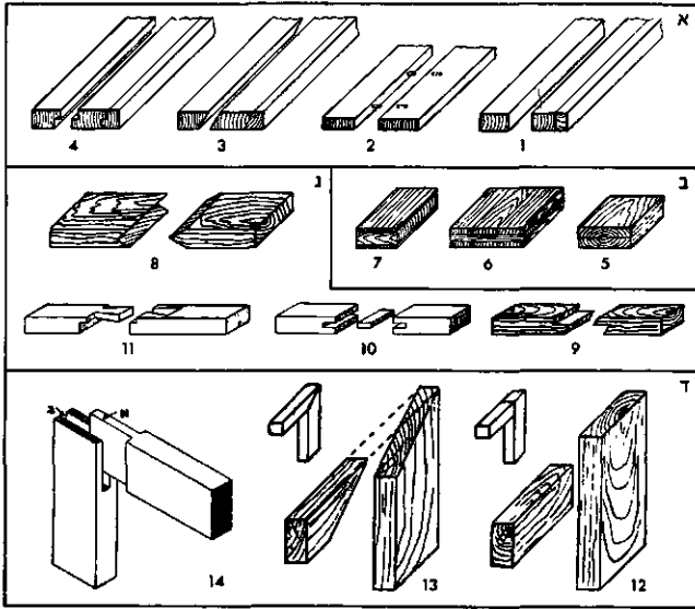
קטברים. א. מחברי רוחב: 1. משק ישר; 2. משק לשון עגולה; 3. משק משופע; 4. משק מדורג. ב. מחברי עובי: 5. כשתי שכבות; 6-7. 3 שכבות; 8. מחברי אורך: 8. קנה בראשית; 9. מנה מדורג; 10. סיוון (עם סיון נפרד); 11. זנב רדור; ד. מחברי זווית: 12. כְּרָע ישר; 13. כְּרָע משופע; 14. עם סיוון (א - סיון; ב - 3/4)
