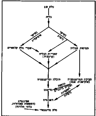
מחזור הסלעים
