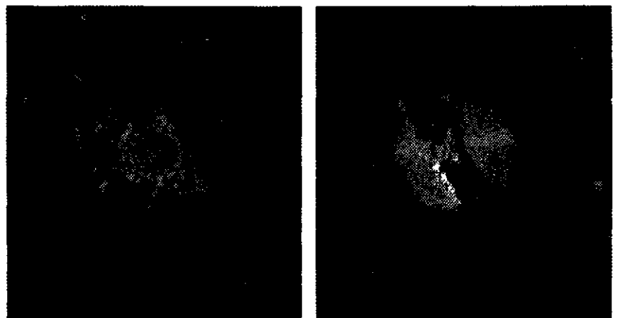
לוח מיון ערפיליות: הטור השמאלי — לוליינית, הימני — לוליינית עם מתג. מלמעלה למטה הזרועות הולכות ונפתחות והכוכבים הנודדים ניתנים יותר להבחנה
