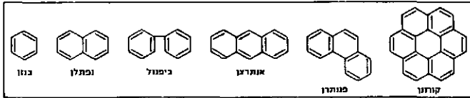
ציור 2: פחמימנים ארומטיים
