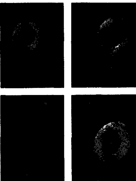
ערפילית פלנטרית כפי שצולמה מבעד למסנני אור המעבירים צבע אחד. למעלה משמאל — ירוק; מימין — אדום; למטה מימין — צהוב; משמאל — כחול
