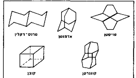
ציור 1: פחמימנים אליציקליים בעלי 2 טבעות ויותר
