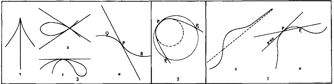
ציור 1. א. המשיק הוא גבול התוחכים PP_1 ; ב. אסימפטוטה, ציור 2. מעגל העיקום (העקמומיות); ציור 3. נקודה מיוחדת של העקום. א. נקודת ספנה; ב. נקודה כפולה; ג. נקודה טרזיבה; ד. חוד
