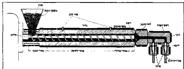
מבנה של מכונת שיחול
