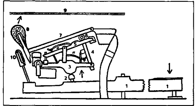
מנגנון של פסנתר, נראנד" מורדני: 1. הקליד; 2. מסוט; 3. מסער; 4. סנוף; 5. סנוף-שנה; 6. נליץ; 7. קת" הפטיש; 8. ראש הפטיש; 9. המיתר; 10. ספר (פטיש הנסוג)
