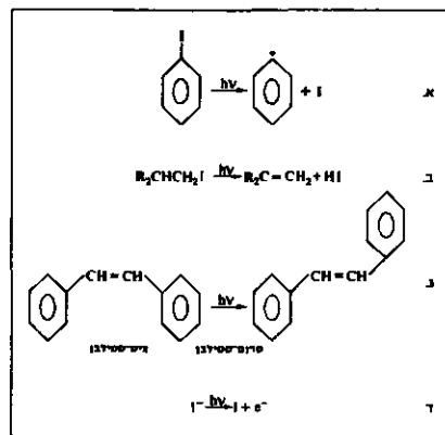
דוגמאות לתהליכים פוטוכימיים חריגותיים. א. פרוק לרדיקלים; פוטוליה של יודרפנון; ב. פרוק לפרודות; פוטוליה של אלקיל הלדים; ג. איזומריזציה; ד. פוטויוניזציה.
