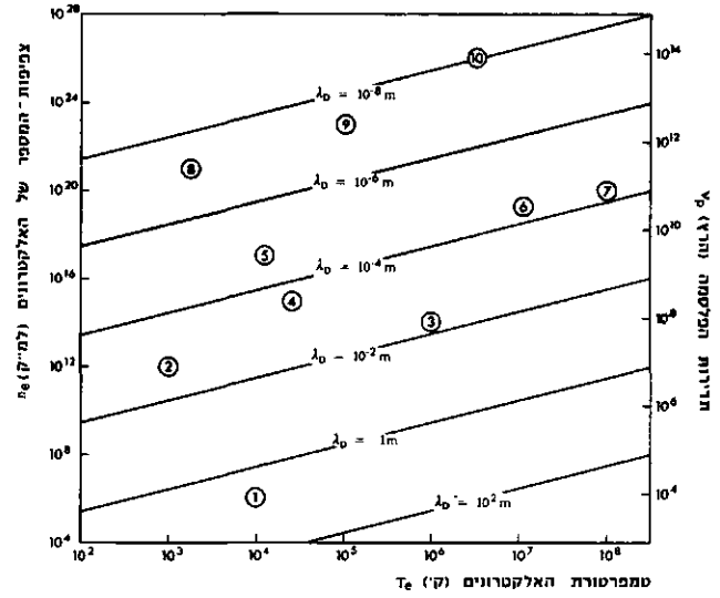
ערכים טיפוסיים לתכונות העיקריות של האלקטרונים בתוך פלסמה: 1. הנו הכי-זכוכי; 2. יונספירה של כד"א (שכבת F); 3. עמדה של השמש (ליד הפוטוספירה); 4. נורות פלואורניות; 5. קשת חשמלית בלחץ נמוך; 6. מתקן Tokamak בפרינסטון, אה"ב (1972); 7. כור סיווג; 8. ייצור מננס-הידרודינמי של חשמל; 9. שפופרת-הלם אלקטרומגנטית; 10. פלסמה מיוצרת ע"י קרני לייזר (ללא רחיסה)
