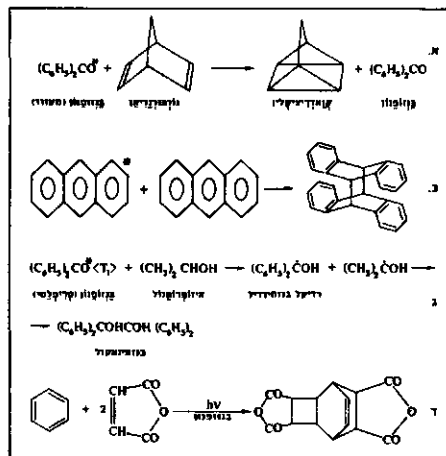
דוגמאות לתהליכים פוטוכימיים דו-פרודתיים. א. הע' כרת אנרגיה מלוחת כאיזומריזציה; ב. פוטודיפרי-זציה; ג. דיפרוויזציה של רדיקל בנוהדירי — התוצר הסופי; ד. פוטויוניזציה.
