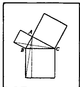
בנייתעור להוכחת משפט פיתגורס (במשולש ישר זווית AB^2 + AC^2 = BC^2 : ABC)
