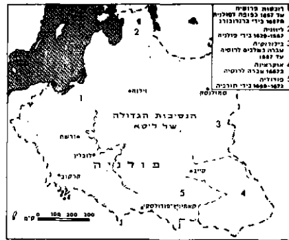
פולניה 1569-1772
