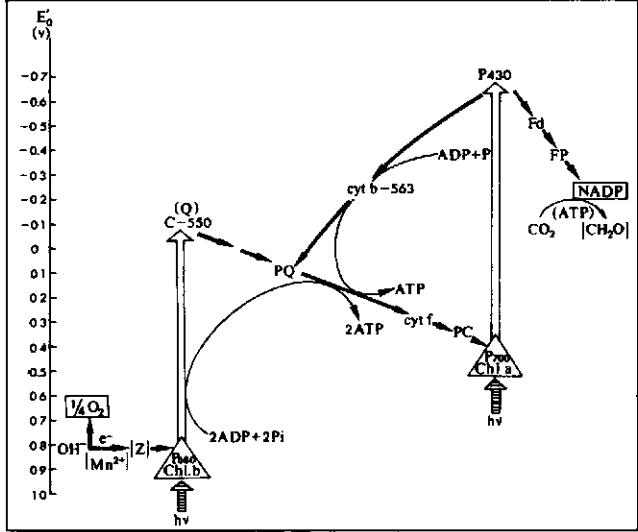
ציור 1: מעבר האלקטרונים והיחסים האנרגטיים במערכת הפוטוסינתטית
