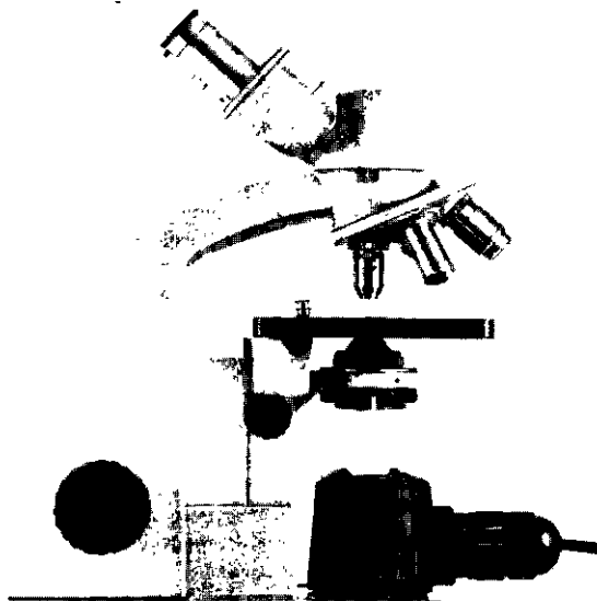
ציור 2ב. המראה החיצוני של מיקרוסקופ מורכב
