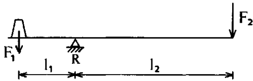
ציור 6. סנוף סכמתי. המשקל F_1 וכוח-ההרמה F_2 יוצרים מומנטים; כוחם השקול מתאזן ע"י התנגות בנקודת-המשען R
