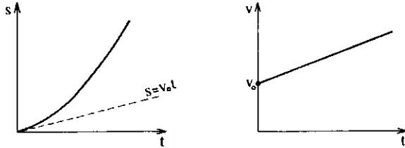
ציור 7. תנועה קווית שוות-תאוצה. מימין: המהירות נרדף באופן ליניארי מערפה ההתחלתי v_0 , משמאל: הדרך מורכבת מתרוסת המהירות ההתחלתית (הישר) ותרוסת התאוצה
