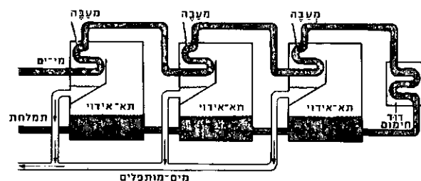
תהליך הזיקוק בהבזקה
