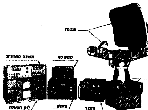
ציור 1. מכ"ם לראטי-ריה
