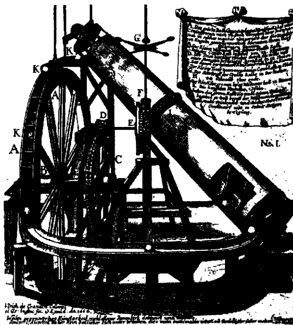
ציור 2. הצעה למכונה תמידית שפורסמה ע"י אולריי פון קראנאר (1864); הספרים לפעולתה רשומים במנילה. — בתוך הצינור נמצא בורג-ארכימדס, המופעל ע"י גלגל-ויטרוביום, שאותו מסובכים הפדורים הנפלים
