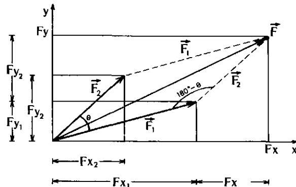
ציור 2. חיבור הרכיבים המתאימים של הוקטורים F_1, F_2 נותן את רכיבי הוקטור השקול F
