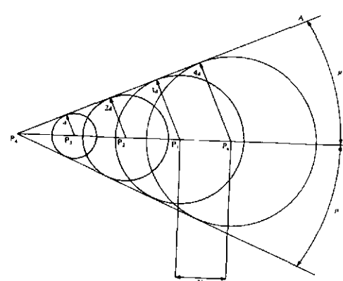
ציור 21. התהוות גלי-הלם על חרוט במהירות על-קולית. הקו P_4-A הוא גל הלם; P_4-P_0 הוא מרכז החרוט של הנללים; a, 2a, 3a, 4a הם רדיוסי הנללים; V הוא מרכז החרוט וסמור הרחיסה; \mu הוא תחום התפשטות הנלים
