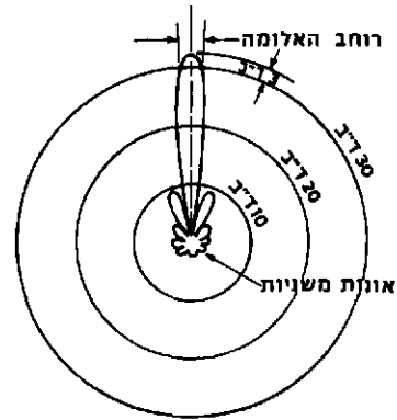
ציור 2. סערך טיפוס של אלומותיהגלים (המשודרים והנקלטים) באנטנה של ספ"ם. הגבף סתאר את התלות בין עוצמתהאות לבין כיוונו
