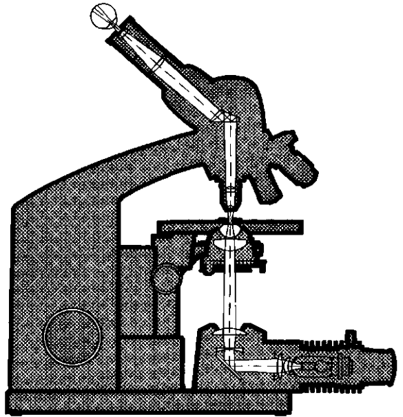
ציור 2א. הטיבנה הפנימי של מיקרוסקופ מורכב ומהלך הקרניים בו
