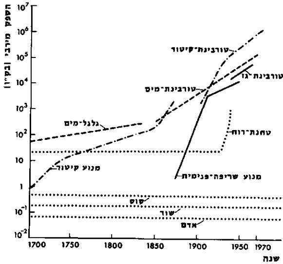
ציור 22. התפתחות מנועים שונים כחסופה המודרנית
