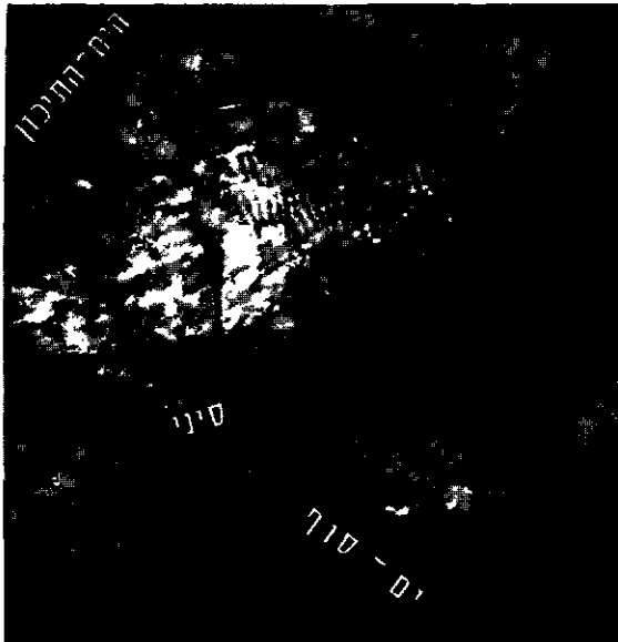
ציור 4. ענני-גלים מעל לא"י (צילום סתור לוויין)
