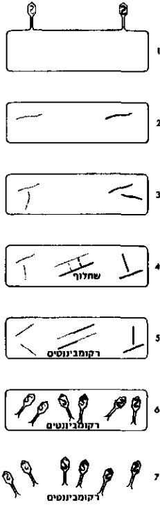
ציור 2. תיאור סכמתי של רקומבינציה בפאנים
