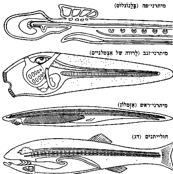
מיתר (|||||) שפופרת עצבים (□) סדקיוזימים ())) מכה נוסף של מיתרנים שונים (ציור סכסתי)
