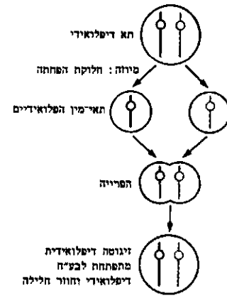
ציור 1. מחזור מיני, המורכב משלבים דיפלואאידים והפלואאידים. כסמכה מצוין רק זוג אחד של כרומוסומים (אחר אפור והשני שחור)
