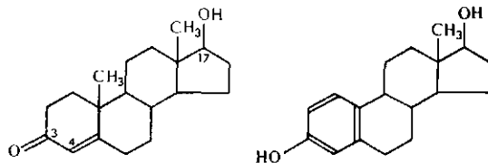
ציור 6. מימין: הורמוני-מין נקבי — אסטראדיול. משמאל: הורמוני-מין זכרי — טסטוסטרון
