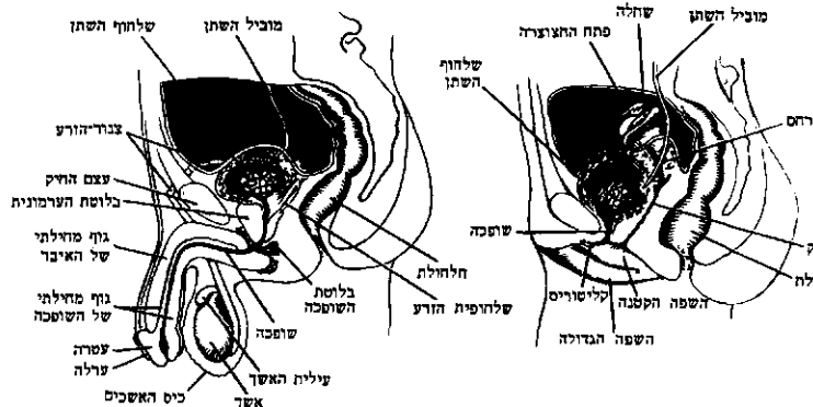
ציור 7. מערכת-המין של אשה וזכר מכוננים. חתך סכמתי
