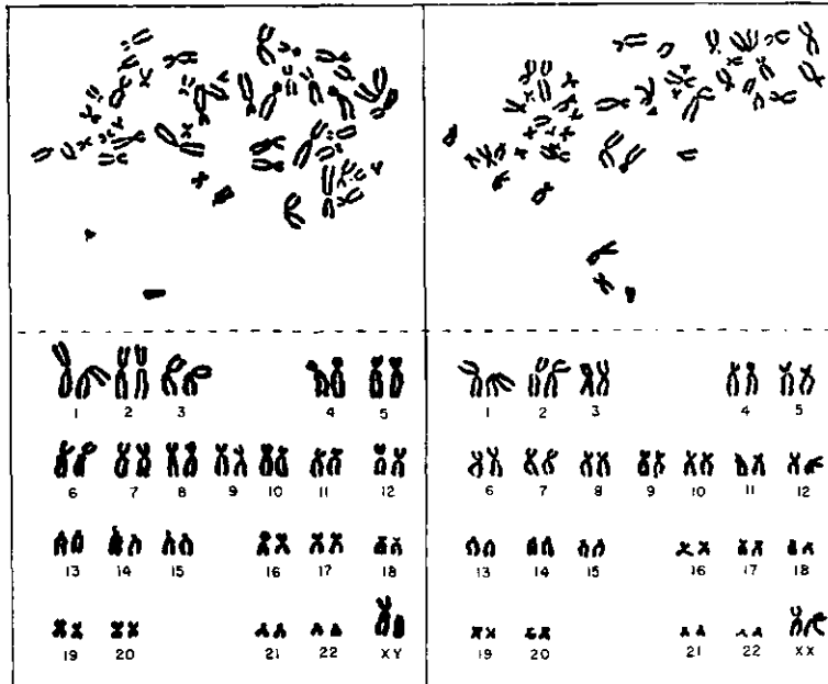
ציור 4. כרומוסומום של האדם: מימין — נקבה; שמאל — זכר. למעלה — הכרומוסומום כפי שצולמו בשלב האמצעי של חלוקת התא; למטה — המונות הכרומוסומום ננדרו וסוננו לזוגותיהם: 22 זוגות אוטוסומום וזוג כרומוסומי-הסין (התחתון מימין בשני הציורים) — הגדלה פי 3000
