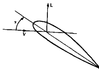
ציור 19. — הזווית בין וקטור המהירות V לבין מיתר הפרופיל; L — וקטור כוח העילוי
