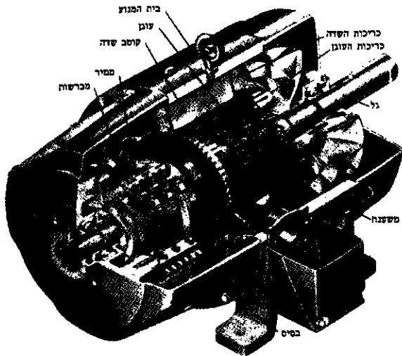
ציור 20. מנוע חשמלי לזרם ישר
