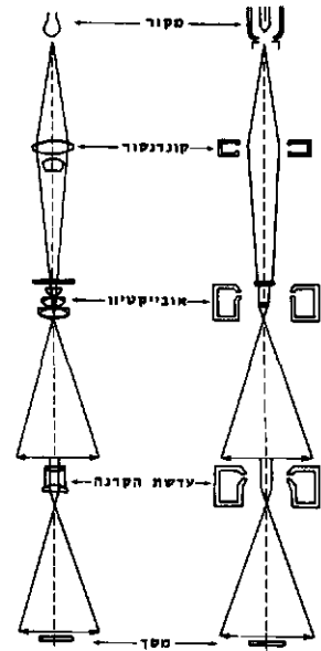
ציור 3. השוואה בין מיקרוסקופ אופטי (משמאל) ומיקרוסקופ אלקטרוני (מימין) — מבחינת הטיבנה ומהלך-הפרניים (בשירי-טוט סודגשת ההקבלה ביניהם)
