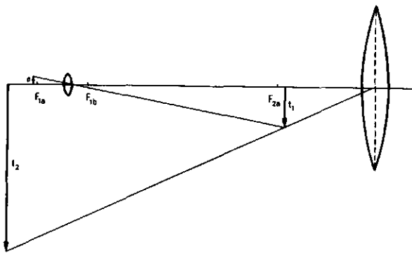
ציור 1. עקרון מהלך הקרניים במיקרוסקופ מורכב: F_{1a}, F_{1b} — מוקדי האובייקטיוו; F_{2a}, F_{2b} — מוקדי האוקולאר ( F_{2b} אינו נראה כשירותוס); e — העצם; t_1 — תמונת-הביניים (הממשית); t_2 — התמונה הסופית (המרוסח)
