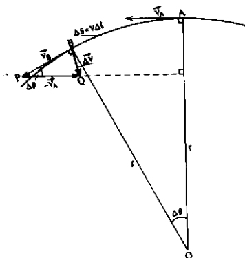
ציור 8. תנועה מעגלית. המהירות בכל סקום ששיקה למעגל, אך כיוונה משתנה; נוצר הפרש-מהירות \Delta v , הניצב למי הירות הקשפית ומכוון אל מרכז-המעגל
