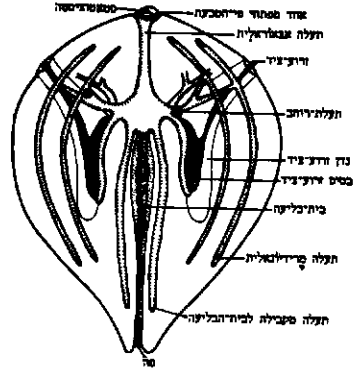
ציור 2. מערכת העיכול של מסרקן (ציור סכמתי)
