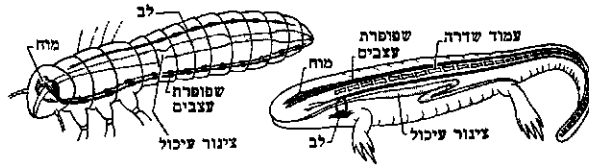
השוואה בין טיפוס מיתרני (סאלאסאנדרה) — ביסיון, לטיפוס חסרי-מיתר (הרק) — בשטאל (ציור סכסתי)
