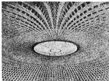
צילום 19. חתרת היכל-הספורט ברוסא (1960), המגנייה מיתרות טרומיות של 600 ס"מ (הארזים: 5, 6, 7, 8, 9, 10, 11, 12, 13, 14, 15, 16, 17, 18, 19)
