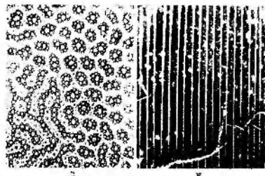
צויר 8. איורים מגנטיים, מודגמים ע"י אבקה מגנטית, נכבש של קובלט. הפישור הפועל במ"א מקביל לצויר ההפסאונדאלי; המישור הפועל במ"ב ניצב ל-19
