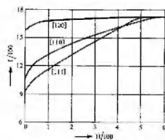
צויר 6. עקומות-מיגנט של נביש אה"ד של ברזל ב-18°C, בשביל כיוונים קריסטלוגרפיים שונים
