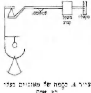
ציור 4. כפיסה מ" מאזניים בעלי כף אחת
