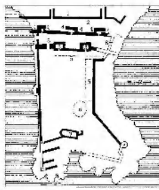
צויר 10. מצודת זלבני בא"י; עתלית — מספט פלדן: 1. חומת היצוגית של החפור; 2. החפור; 3. מגדלים כוכבי-צורה; 4. שני מ" ששייכים למבצרי קוהביצורים חתי; 5. מבנים סמורים; 6. עממית, אצורי היצוגית; 7. אולם קטור; 8. שערים
