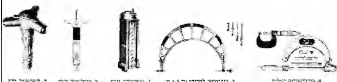
א. מיקרומטרים חוטים ב. מיקרומטר למדידה עד 1.5 מ"מ ג. מיקרומטר נקמת ד. מיקרומטר זווית ה. מיקרומטר זווית
