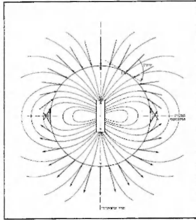
ציוור 2. עצמת השדה F בנקודות שונות על-פני כדור סמוגנס בצורה אחידה, החתך עובר דרך ריזארד של השדה המגנטי. בנקודה L צוינה הווית I — כיוון לאופק המסומן
