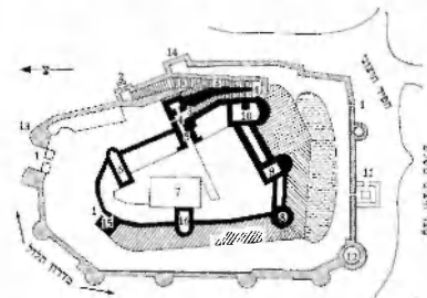
צויר 8. גדר רה שווליה — מבצר זלכני בסוריה מקרא למצוית שטחתי לצויר: 1. משפטים; 2. שער ראשי חיצוני; 3. עלות מכוסה נג לשער הראשי הפנימי; 4. פיתולים חשופים לזר; 5. שער ראשי פנימי; 6. שער ראשי פנימי; 7. אולפית; 8. שער סטרי המבצר; 9. מיוון עקביות; 10. מבנה סאולר מתקופת הסוסלמית; 11. בניינים פאחרים מתקופת הערבית; 12, 13, 14. בניינים קורמים לפעוים התיקריים
