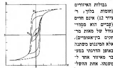
ציור 11. עקומת-החלש בטמפרטורה ערכים שונים של שדות מנספטיים
