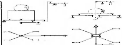
צור 8. מאזני-כדור משקולת משאול כבדים, משאול קלונות-רבנת וכד' (למשלה — מכס מו הצור, למטה — מכס מלמעלה)
