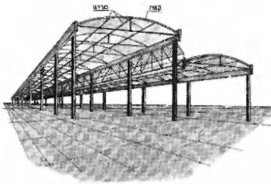
צויר 7. סכנה לתעויה: מערכת קשתות ומרישים מפלדה
