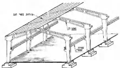
צויר 6. אולם לתעויה: שלד של סכנרות מסבך; סוויין
