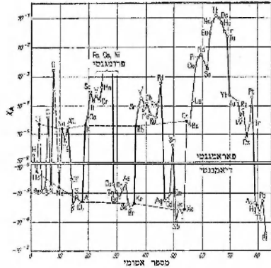
ציר 4. הסוספטיביליות האטומית של היסודות בטמפרטורת החדר
