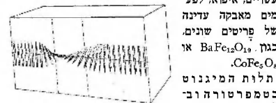
ציור 12. סכמת של הגבול (חומי-בלוך) המפריד בין שני איזורים
