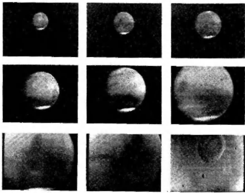
ציון 4. התצלומים מארינו UV בהתמרחותה אל המאדים, הצילומים נעשו בתאריכים 29-31 ביולי 1968. הצילום הראשון נעשה מסרח של 1,241,260 ק"מ מן המאדים, ואילו האחרון, שפי ניוו הבהינו במשך שטחו של 883 ק"מ - מסרחו של 3,600 ק"מ. השם המפור הוא כיפת-הקוטב הדרומית
