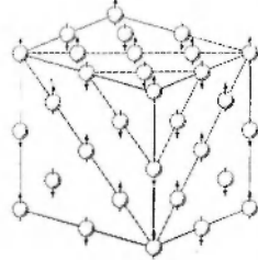
ציור 14. סבירה המגנטית של היונים MnO_2 Mn 2+
