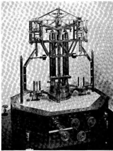
המאזניים המדוייקים ביותר שנבנו עד עתה להשוואת משקלות סטנדרטיות של ק"ג אחד, הם נמצאים במעבדה הלאומית במאנצ'סטר, דרום השקילה 1:1 מיקרוגרם
