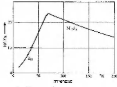
ציור 13. דמוספטיביליות המולקולרית של נביש אחיד של MnF (כבול) מפינס ציור הסטראונגולי של הנביש
