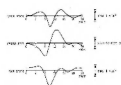
ציור 7. שינויים יומיים במרכיבים המגנטיים; רישום צפוני שעורר במשך יום "שטם"
