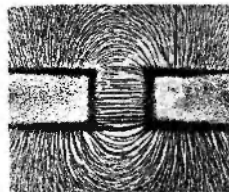
צויר 2. השדה המגנטי בכביכת שני קטבים מגנטיים הרוכים בסימנם
