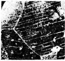
ציור 9. איזורים מגנטיים, מורמים ע"י אפקט מנגנטי, באיזור הנכבול בין שני נבישנים של ברזל חמרי
