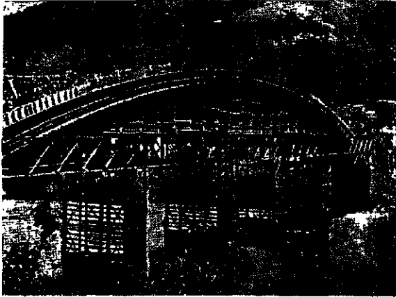
24. תמיכות עץ בכניית קשת בסוף מוזיון (סיפת-הקשת 186 מ')— בגשר ריו דאסיאנטאס בכראזיל
