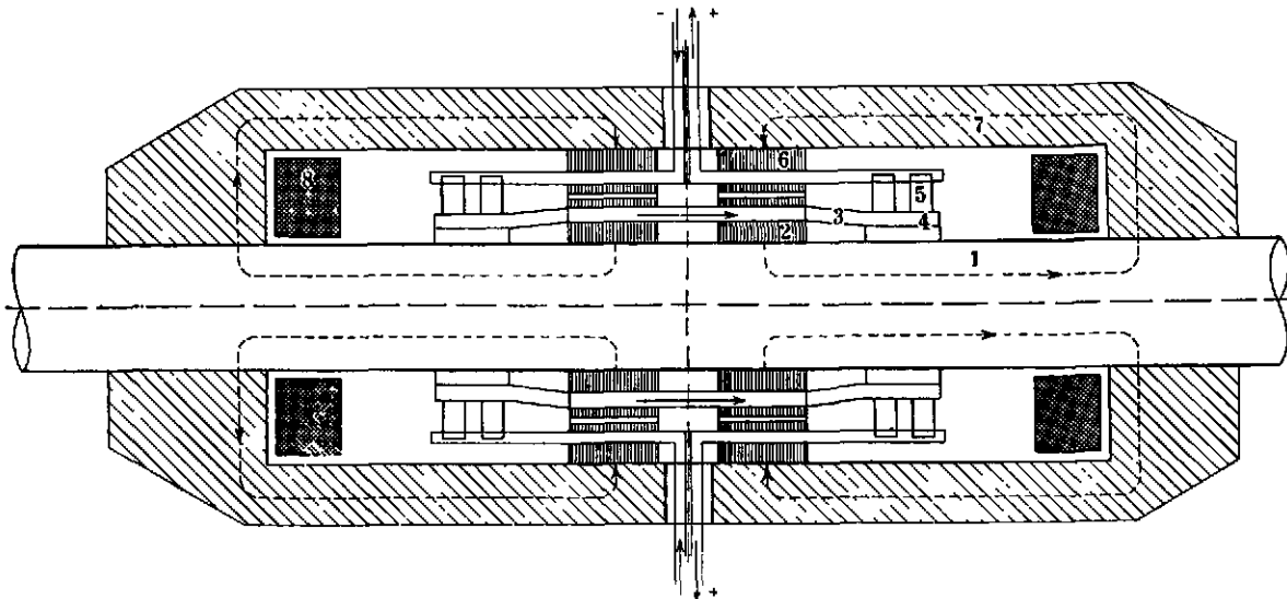
ציור 3 נגראטור. מכונה הטרופולארית (סקמה)
