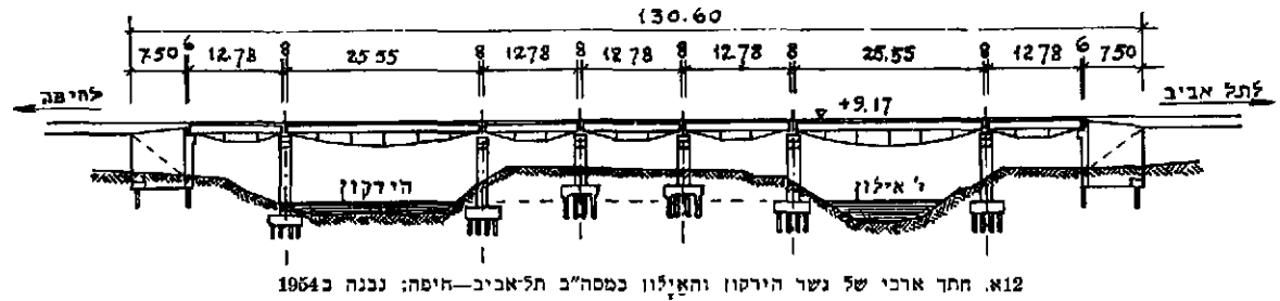
102. חתך ארכי של גשר הירדן והאילון במס"ב תל-אביב—חיפה; נבנה ב-1964
