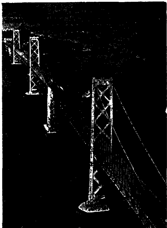
18 גשר סאן-פראנציסקו-אסקלנר מעל למפרץ סאן-פראנציסקו האורך הכללי — 18¼ ק"מ החלקים העיקריים — זוג נשרים תלויים, שסיפחת כל אחד מהם 704 מ' (אורך הוונ התלוי — 2,820 מ'), ונשרי-זיויים (ר' ציור 14 ב)
