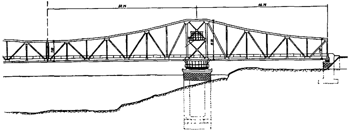
20. נשר סובב מעל תעלת סואץ: האורך הכללי—210 מ', אורך 2 הורעות הסיככות—112.5 מ'
