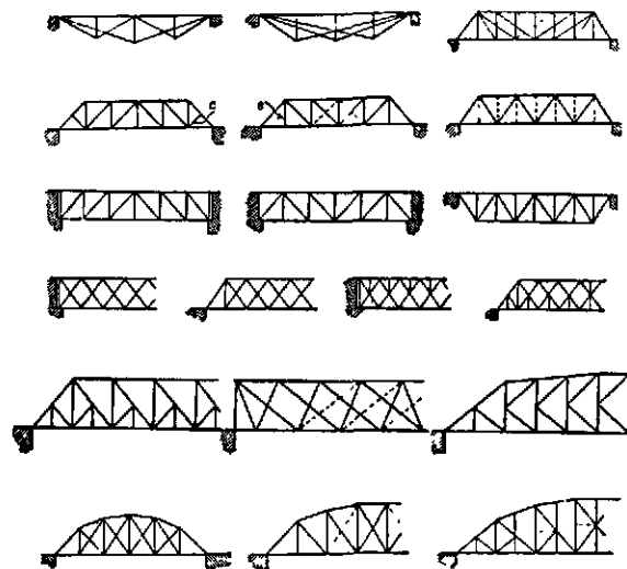
11 טיפוסים שונים של גשרי-מיסבכים
