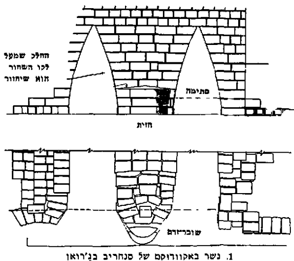
1. גשר באקוודוס של סנחריב בנ'רוואן
