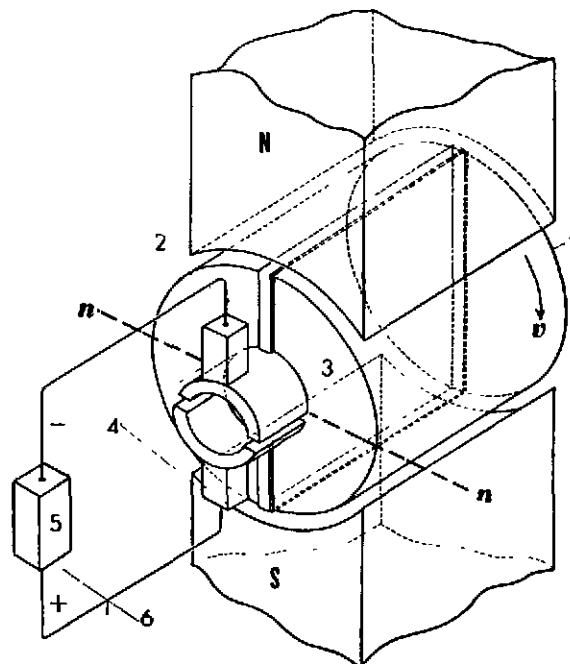
ציור 4. נגראטור. מכונה הטרופולארית (סקמה)
