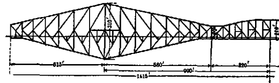
14 א גשר זיזיים מעל לנהר סאו־לורנס בקאנארה (ניקרוויבק)
