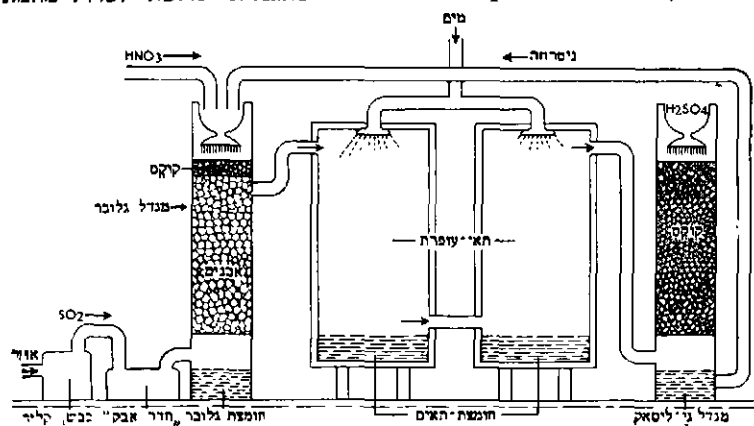
ציור 1 תהליך תאי-העופרת (סכמה)
