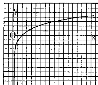
ציור 2 הצגה גראפית של הפונקציה הלוגאריטמית y=\ln x (צלע-הטרובע = \frac{1}{2} )
