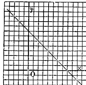
ציור 1 הצגה גראפית של הפונקציה x+y=4 (צלע-הטרובע = \frac{1}{2} )
